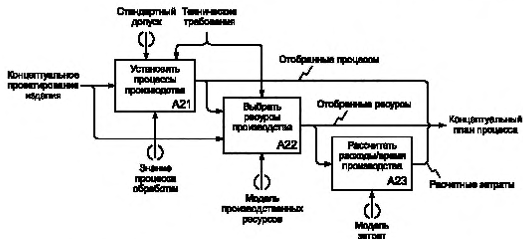
Рисунок В.8 — Функциональное разбиение концептуального планирования процесса
