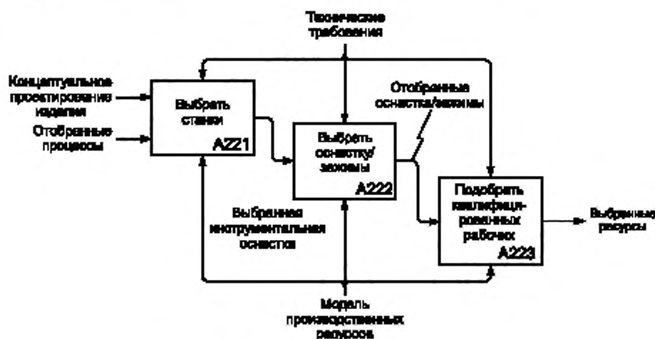
Рисунок В.9 — Выбор производственных ресурсов
