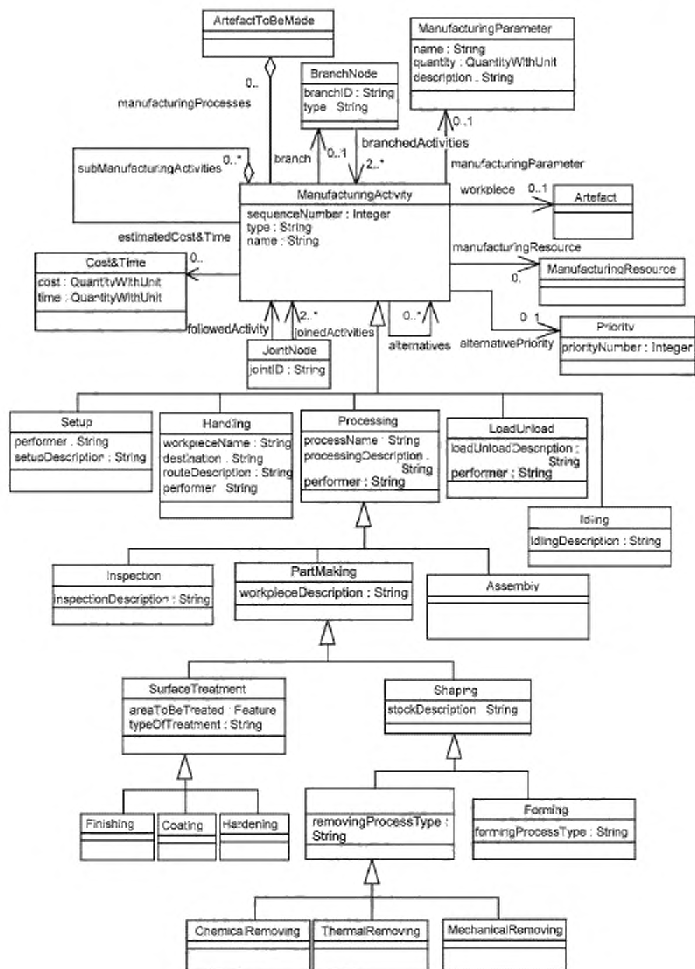
Рисунок В.10 — Диаграмма класса ManufacturingProcess
