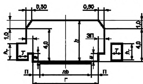
а — при отсутствии разделительной полосы
