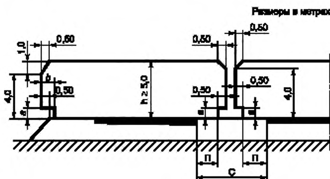
в — при наличии опор на разделительной полосе и ограждений на дороге
