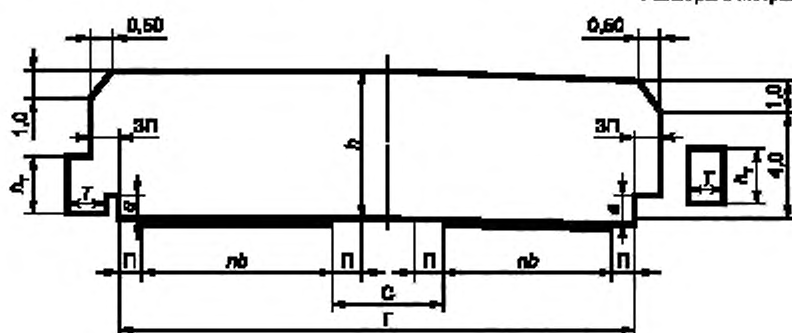
б — с разделительной полосой без ограждений
