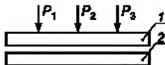
Рисунок 5 — Схема приложения ряда сил вместо одной P = P_1 + P_2 + P_3
