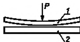
Рисунок 4 — Схема возможной деформации прокладки
