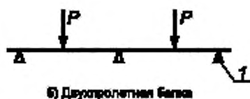
Рисунок 1 — Схемы приложения сосредоточенных нагрузок
