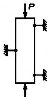
Рисунок 13 — Схемы закрепления стоек при испытании
