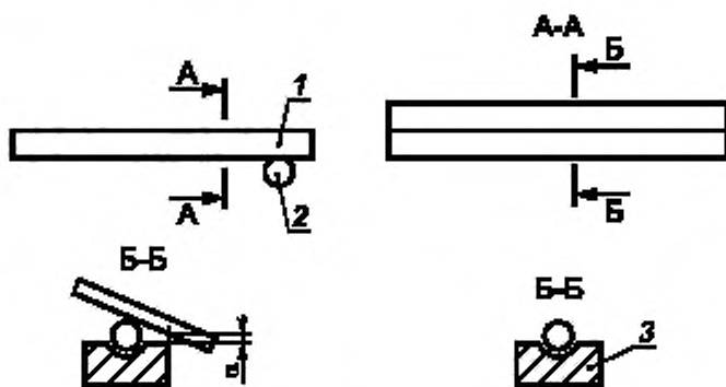
1 — щит; 2 — опора; 3 — седло опоры; a — зазор между щитом и седлом опоры
