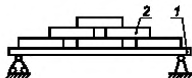
1 — испытательный образец; 2 — штучные грузы
