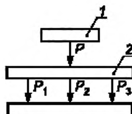
Рисунок 6 — Схема передачи нагрузок с помощью траверсы
