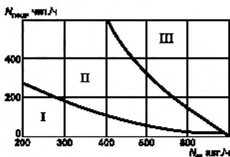
I — нерегулируемые наземные переходы; II — регулируемые наземные переходы; III — внеуличные переходы (надземные и подземные)
