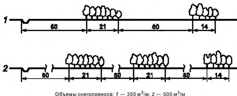
Рисунок 2 — Схемы снегозащитных насаждений для объемов снегоприноса более 300 м 3 /м
