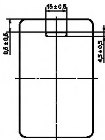
Рисунок В.1 — Щелевое отверстие для портретной ориентации
