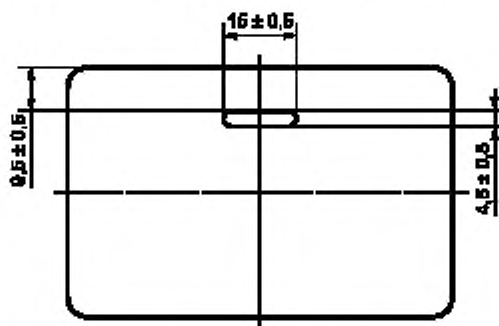
Рисунок В.2 — Щелевое отверстие для пейзажной ориентации
