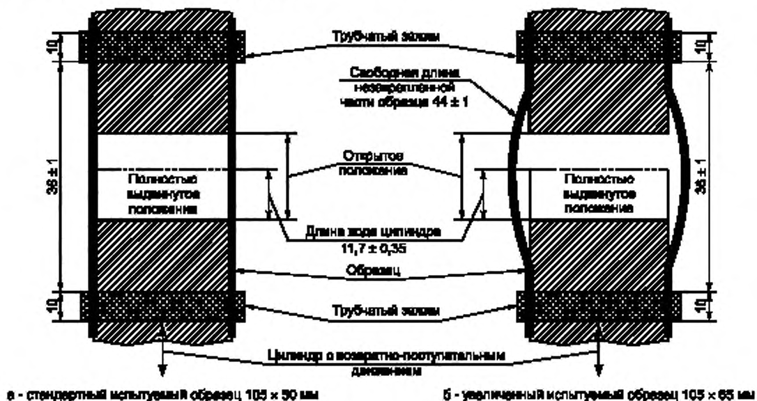
Рисунок 1.2 — Схема заправки образцов для испытания
