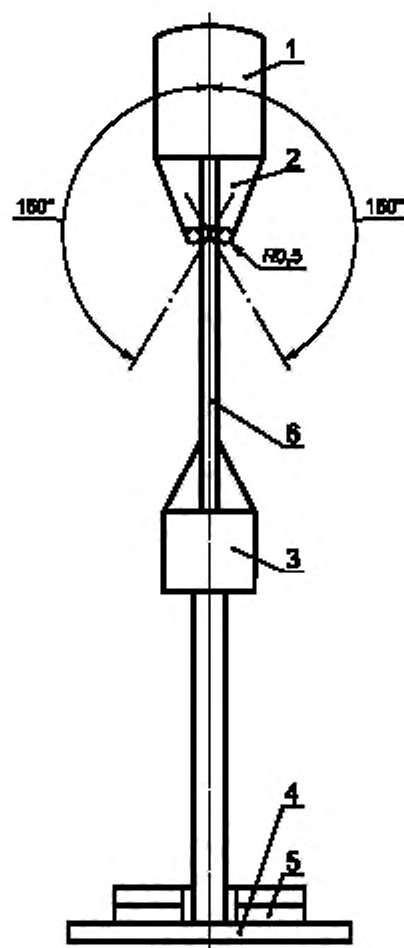
1 — верхний подвижный зажим; 2 — губки определенного радиуса кривизны; 3 — нижний подвижный зажим; 4 — площадка; 5 — дополнительный груз; 6 — испытуемый образец
