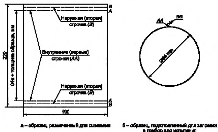
Рисунок 1.4 — Форма образца для испытания на скручивание/изгиб
