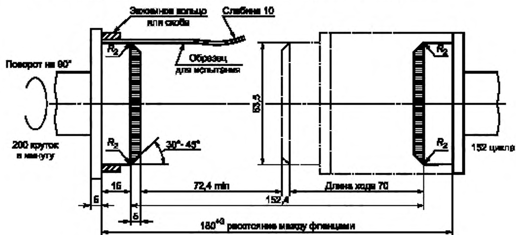
Рисунок 1.3 — Схема прибора для испытаний на скручивание/изгиб
