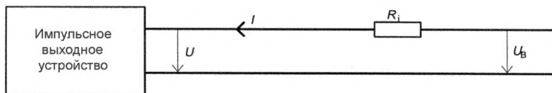
Рисунок Е.2 — Испытательная схема импульсного выходного устройства
