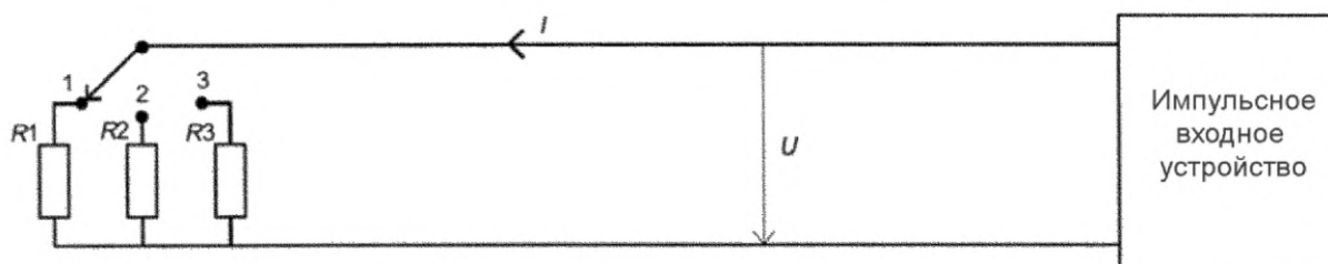
Рисунок D.1 — Испытательная схема импульсного входного устройства
