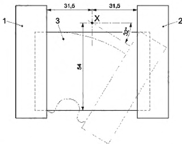
Рисунок 1 — Вид сбоку на образец для испытаний в V-образных зажимах (допуски на размеры даны в тексте)
