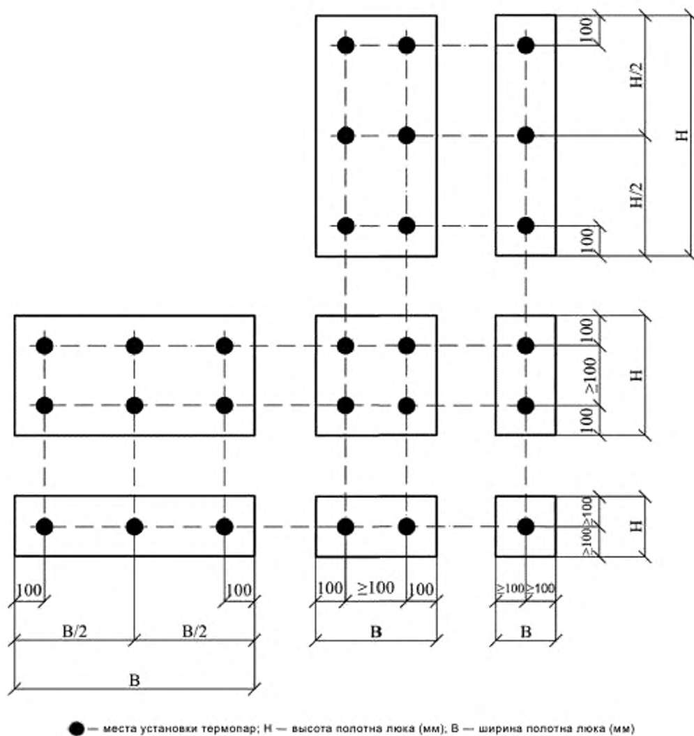
Рисунок А.5 — Схемы установки термодатчиков на необогреваемой поверхности люков площадью полотна, не превышающей 0,25 м 2
