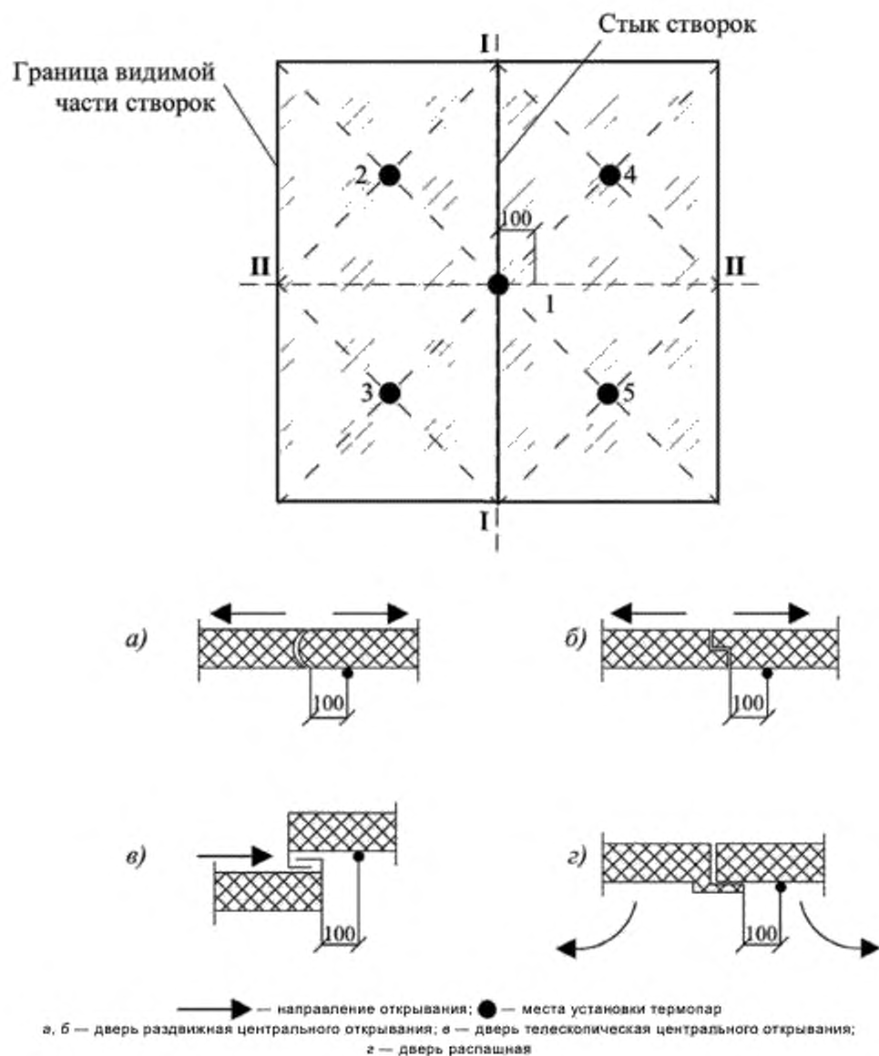
Рисунок А.4 — Схема установки терморпар на необогреваемой поверхности двухстворчатой двери
