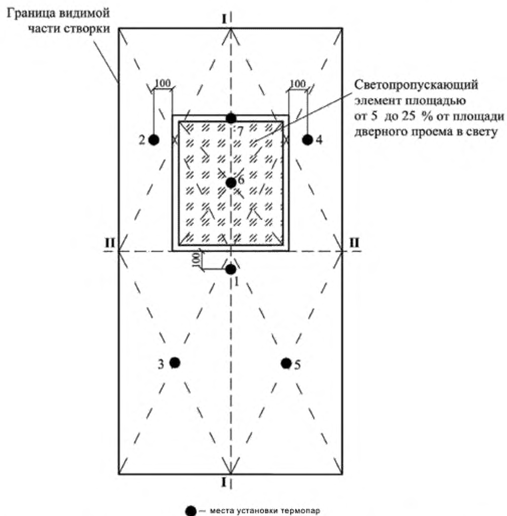
Рисунок А.2 — Схема установки термопар на необогреваемой поверхности створки односторчатой распашной и горизонтально-раздвижной двери бокового открывания со светопроницающим элементом створки свыше 5 % до 25 % от площади дверного проема в свету
