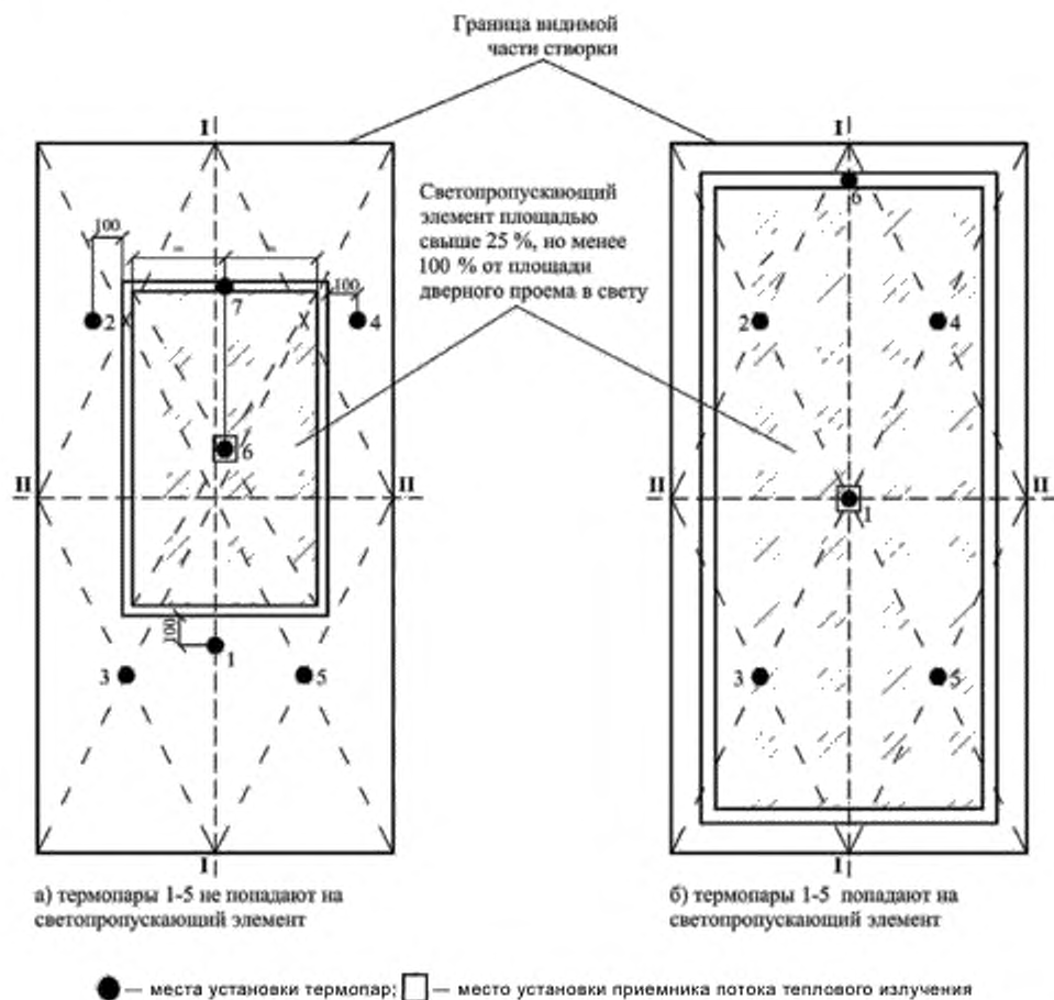
Рисунок А.3 — Схема установки термомпар и приемника потока теплового излучения на необогреваемой поверхности створок одностворчатой распашной и горизонтально-раздвижной двери бокового открывания со светопроницающим элементом створок свыше 25 %, но менее 100 % от площади проема в свету
