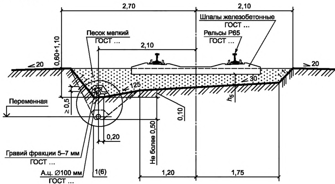
Тип 2. Конструкция земляного полотна и верхнего строения пути на планируемой территории с заглубленной балластной призмой
