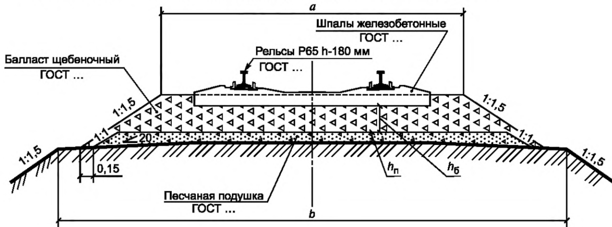
Тип 1. Конструкция на незастроенной территории с открытой балластной призмой
