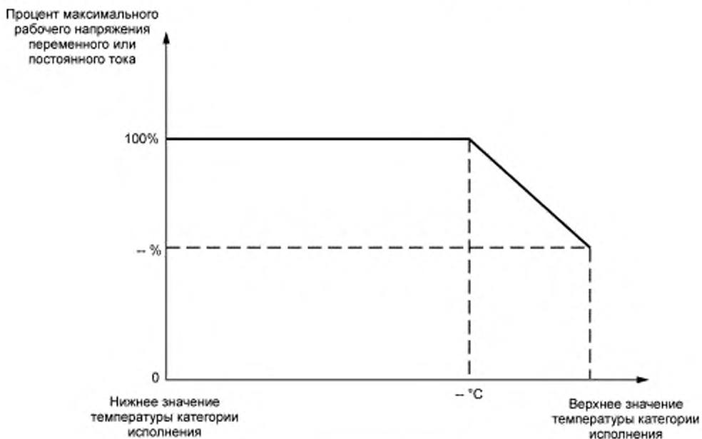
Рисунок 1 — Максимальные рабочие напряжения переменного или постоянного тока
