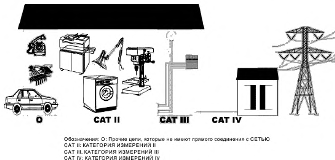
Рисунок AA.1-Примеры идентификации размещения измерительных цепей
