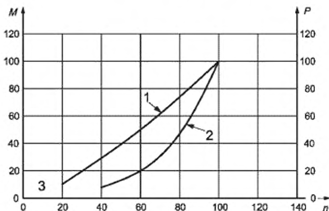
1 — крутящий момент E4; 2 — мощность E3; 3 — холостой ход двигателя в интервале 0—20 % от объявленной частоты вращения
