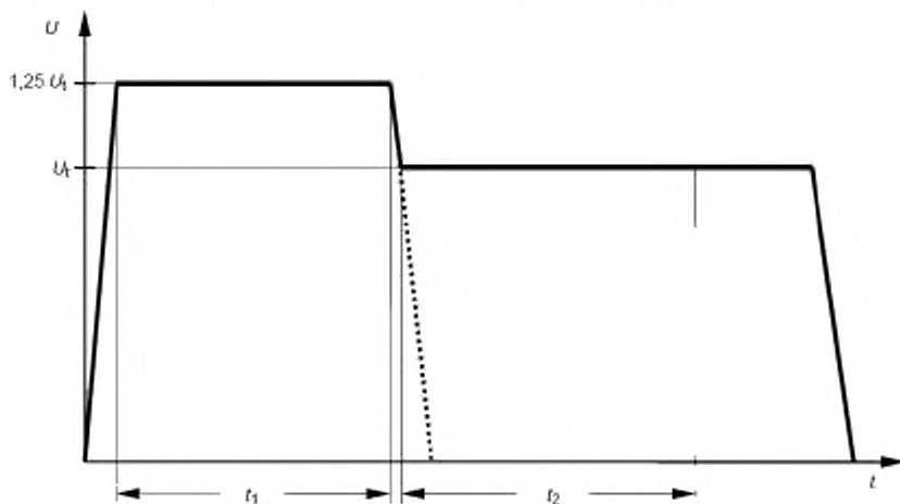
Рисунок 1 – Испытательное напряжение
