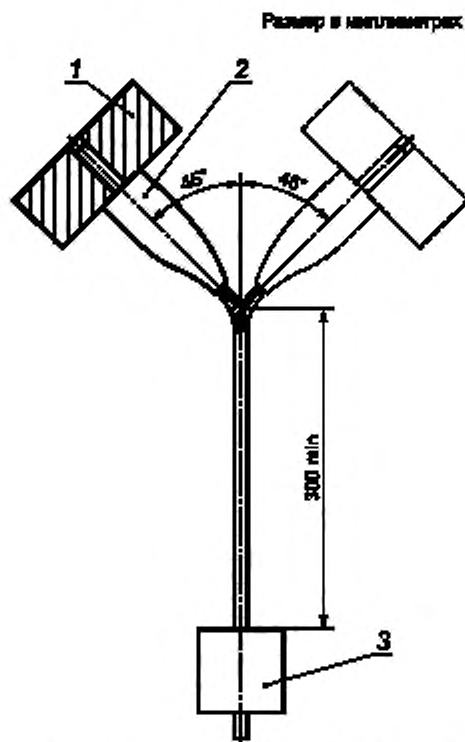
Рисунок 20 — Установка для испытания узла крепления шнура
