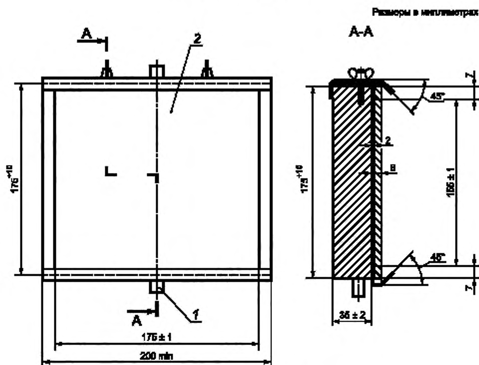
Рисунок 23 — Ударный элемент
