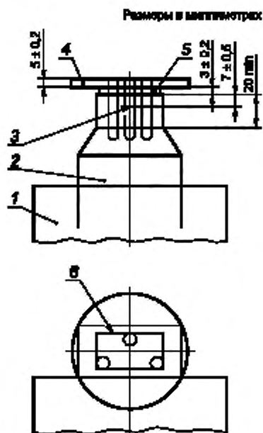
1 — нагревательный элемент; 2 — металлическая часть (деталь); 3 — термометр; 4 — изолирующая плита; 5 — прокладка; 6 — контур вилки
