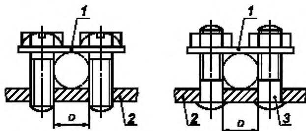
1 — прижимная пластина; 2 — неподвижная деталь; 3 — шлифка. D — место расположения проводника
