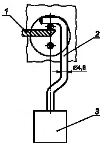
Рисунок 14 — Установка для испытания трубчатых штырей
