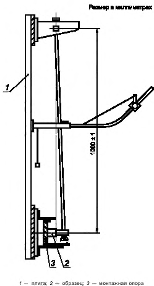
Рисунок 22 — Установка для проверки механической прочности соединителей
