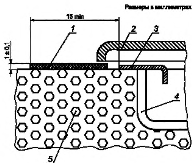
Рисунок 31 — Устройство для испытания крышек и закрывающих пластин (накладок)
