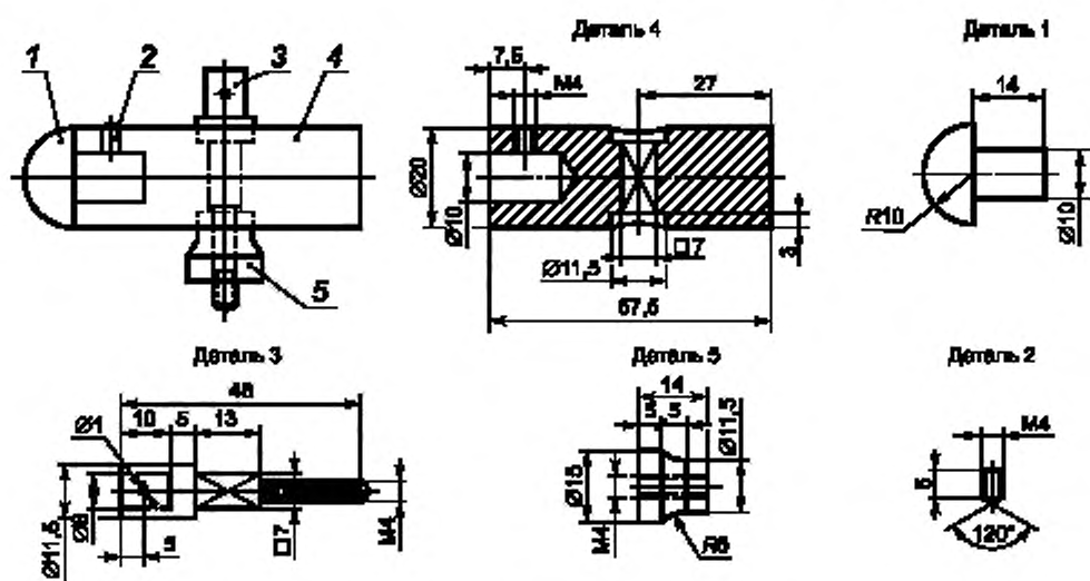
Рисунок 23 — Ударный элемент
