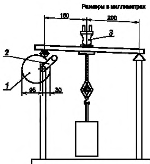
Рисунок 20 — Установка для испытания узла крепления шнура
