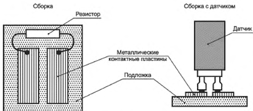
Рисунок 3 — Сборка для проверки сопротивления
