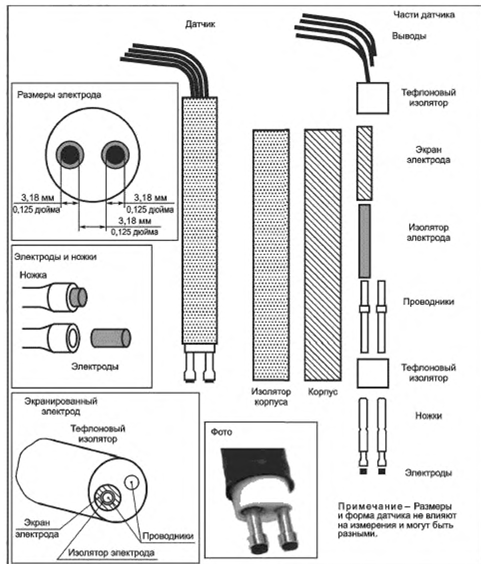
Рисунок 1 — Конфигурация двухконтактного датчика
