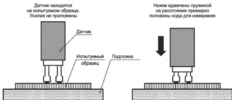
Рисунок 4 — Сжатие пружин при измерении
