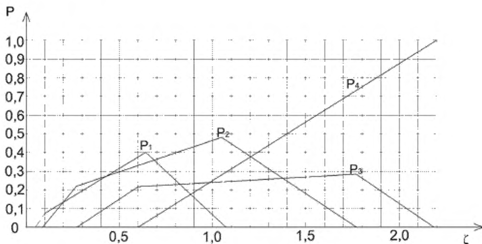
Рисунок 4.1 — Вероятности различной степени разрушения здания (сооружения) и повреждения технологического оборудования в зависимости от величины обобщенного показателя устойчивости, \xi_{зд}(\xi_{ТО})
