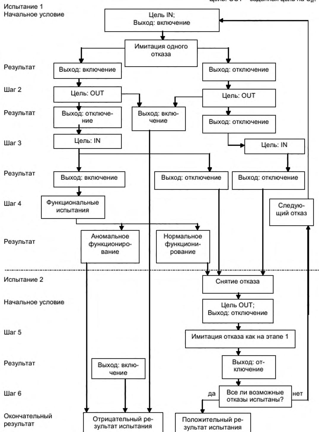
Рисунок А.2 – Последовательность испытаний для ОБД-S
