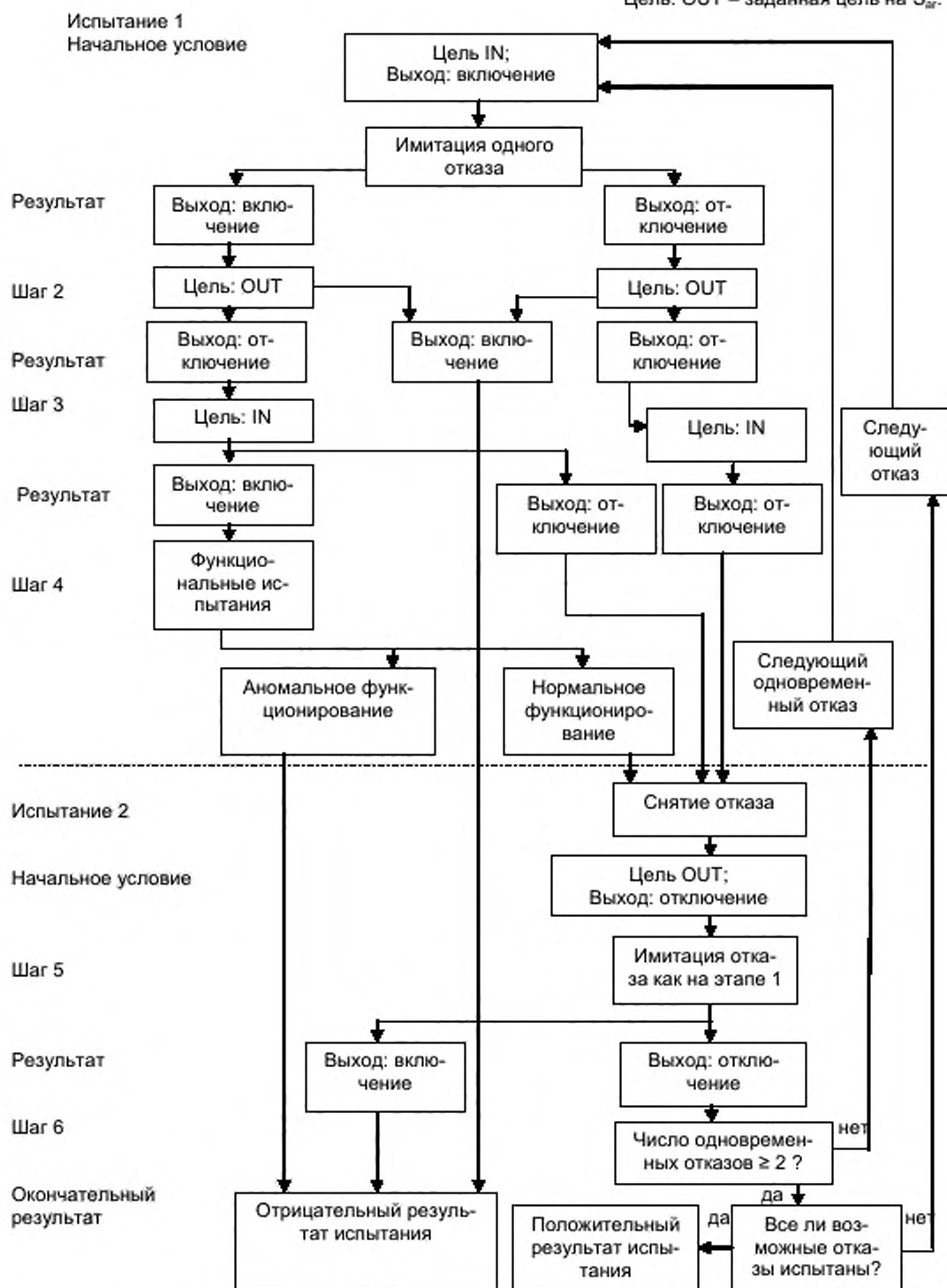
Рисунок А.3 – Последовательность испытаний для ОБД-М
