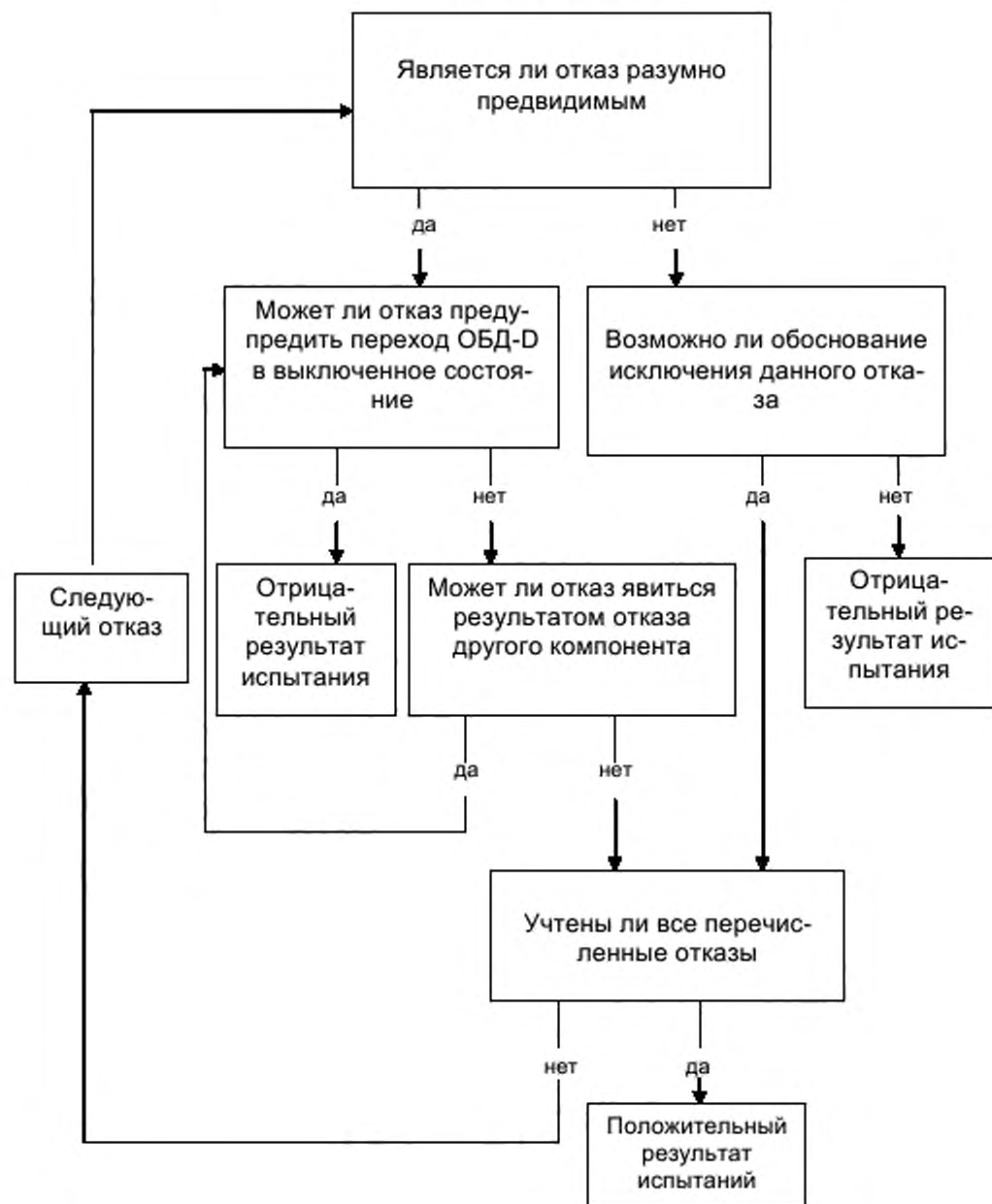
Рисунок А.1 – Оценка отказа для ОБД-D
