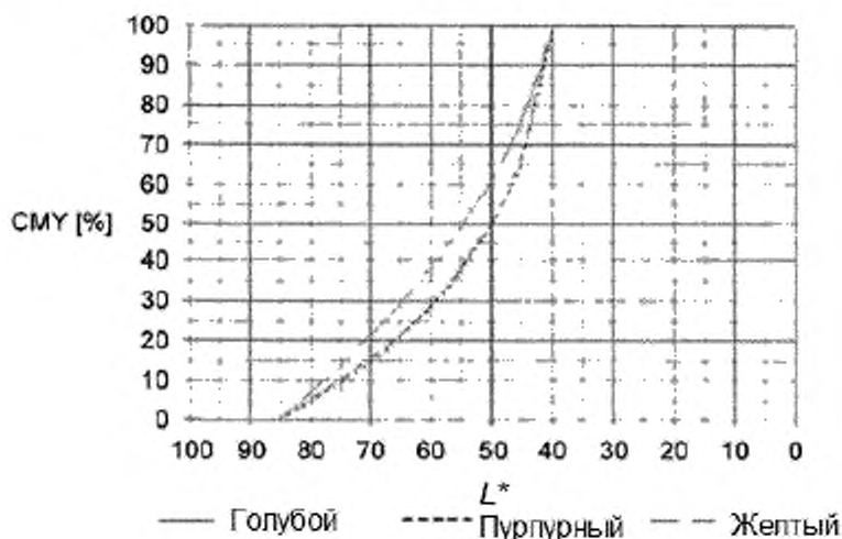
Рисунок В.3 — Пример кривых баланса по серому
