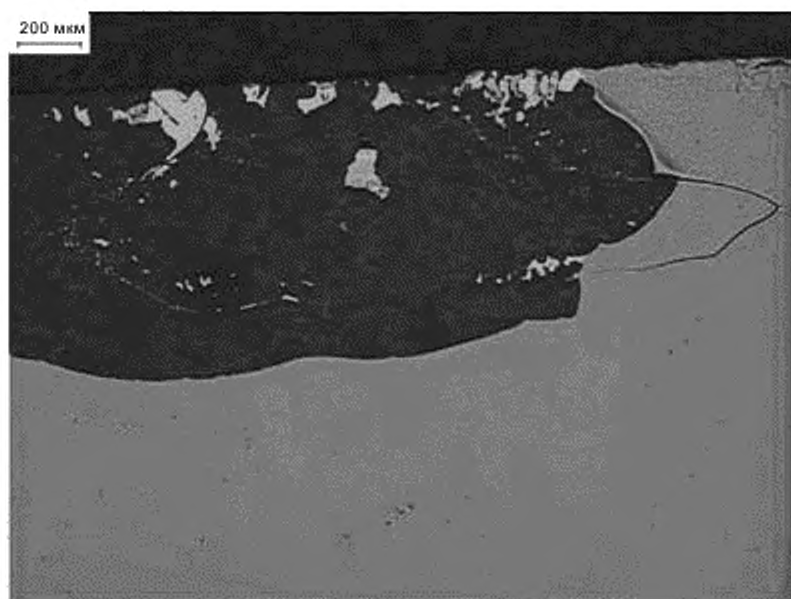
Рисунок А.14 – Отслаивание
