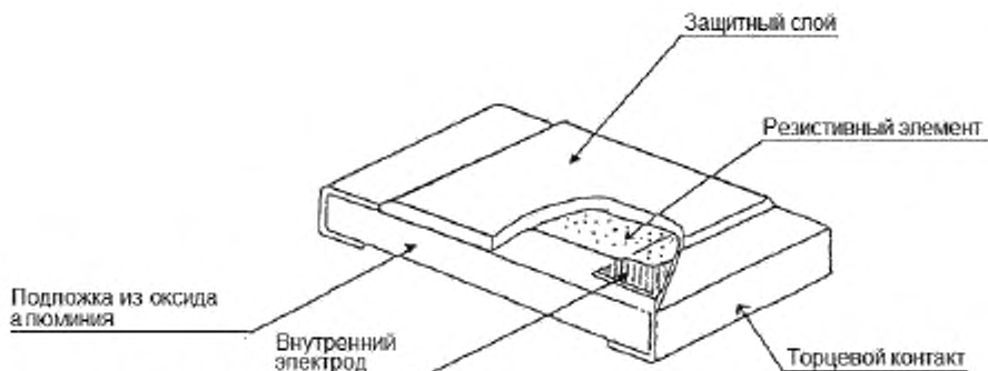
Рисунок 2 – Конструкция прямоугольного безвыводного резистора
