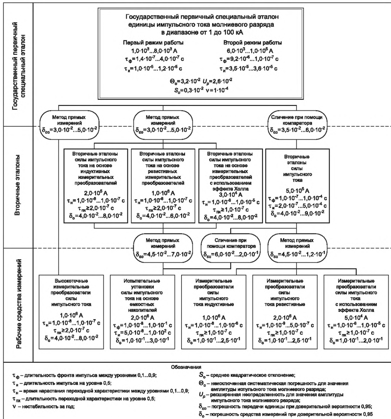
Рисунок А.1 — Государственная поверочная схема для средств измерений силы импульсного тока молниевое разряда в диапазоне от 1 до 100 кА
