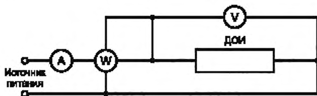
Рисунок А.2 — Рекомендуемая схема определения коэффициента мощности ДОИ
