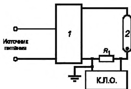
1 — испытуемый ПРА; 2 — номинальная лампа, К.Л.О. — осциллограф
