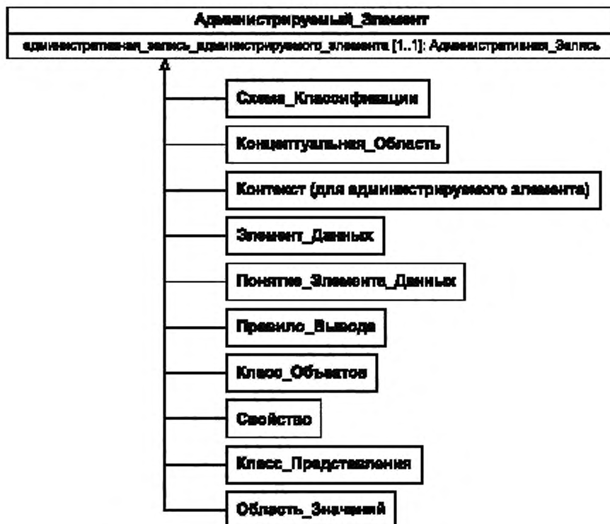
Рисунок 2 — Типы Администрируемых элементов (Сог.1:2004)
