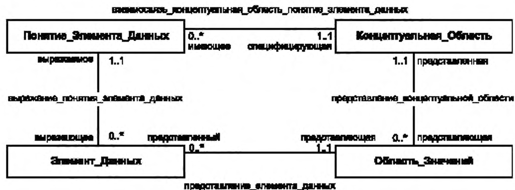
Рисунок 3 — Общий вид метамодели
