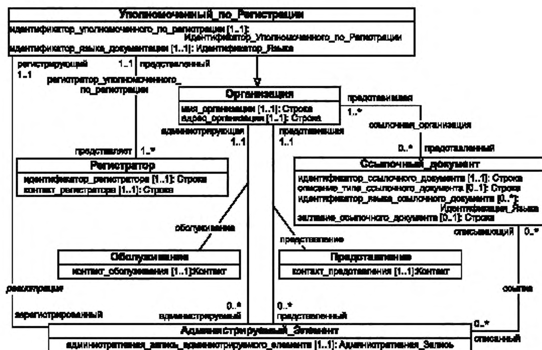
Рисунок 4 — Область Администрирования и Идентификации метамодели
