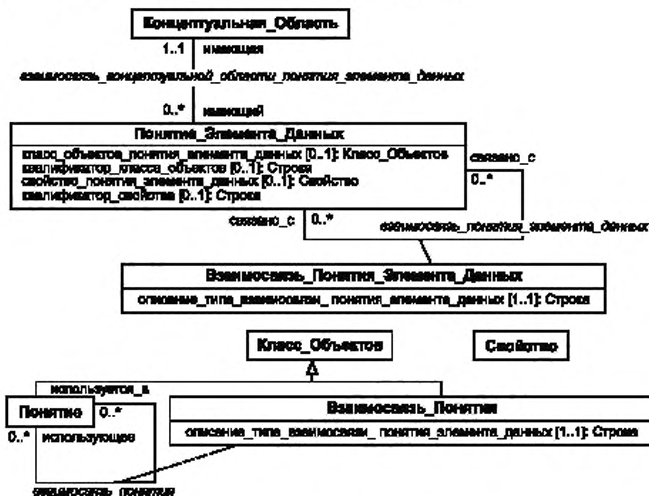
Рисунок 8 — Область Понятий Элементов данных метамодели (Cor.1:2004)
