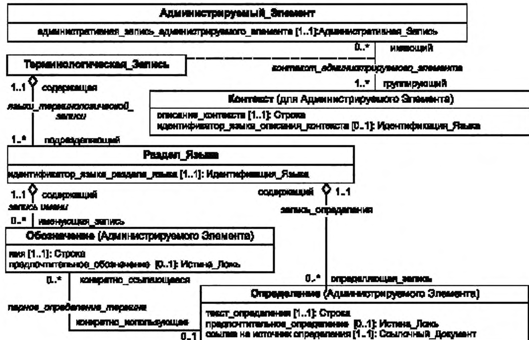
Рисунок 6 — Область Наименования и Определения метамодели (Cor.1:2004)
