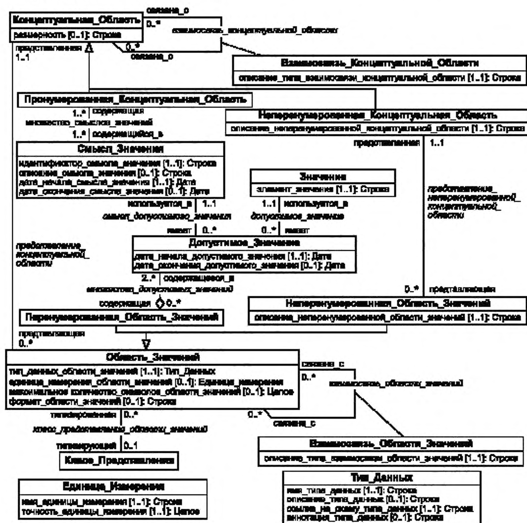
Рисунок 9 — Концептуальная Область и Область Значений
