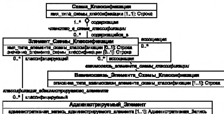
Рисунок 7 — Область классификации метамодели (Cor.1:2004)
