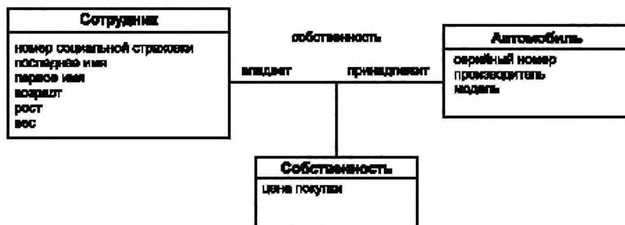
Рисунок В.1 — Пример моделирующей диаграммы
