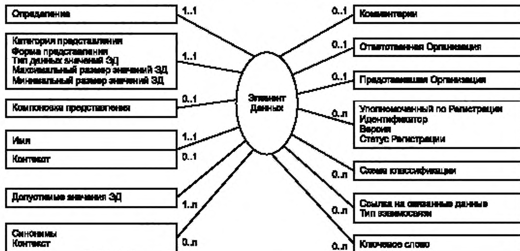
Рисунок С.1 — Базовые атрибуты элементов данных
