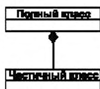
Рисунок В.9 — Нотация для составной агрегации
