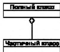
Рисунок В.8 — Нотация для агрегации
