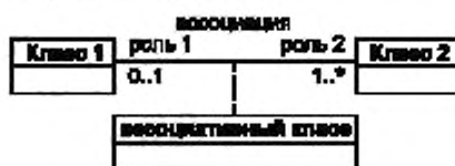
Рисунок В.6 — Нотация для ассоциативного класса
