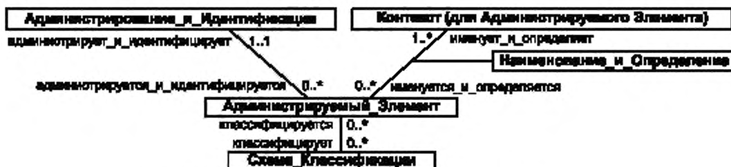
Рисунок 1 — Общие для всех Администрируемых элементов возможности
