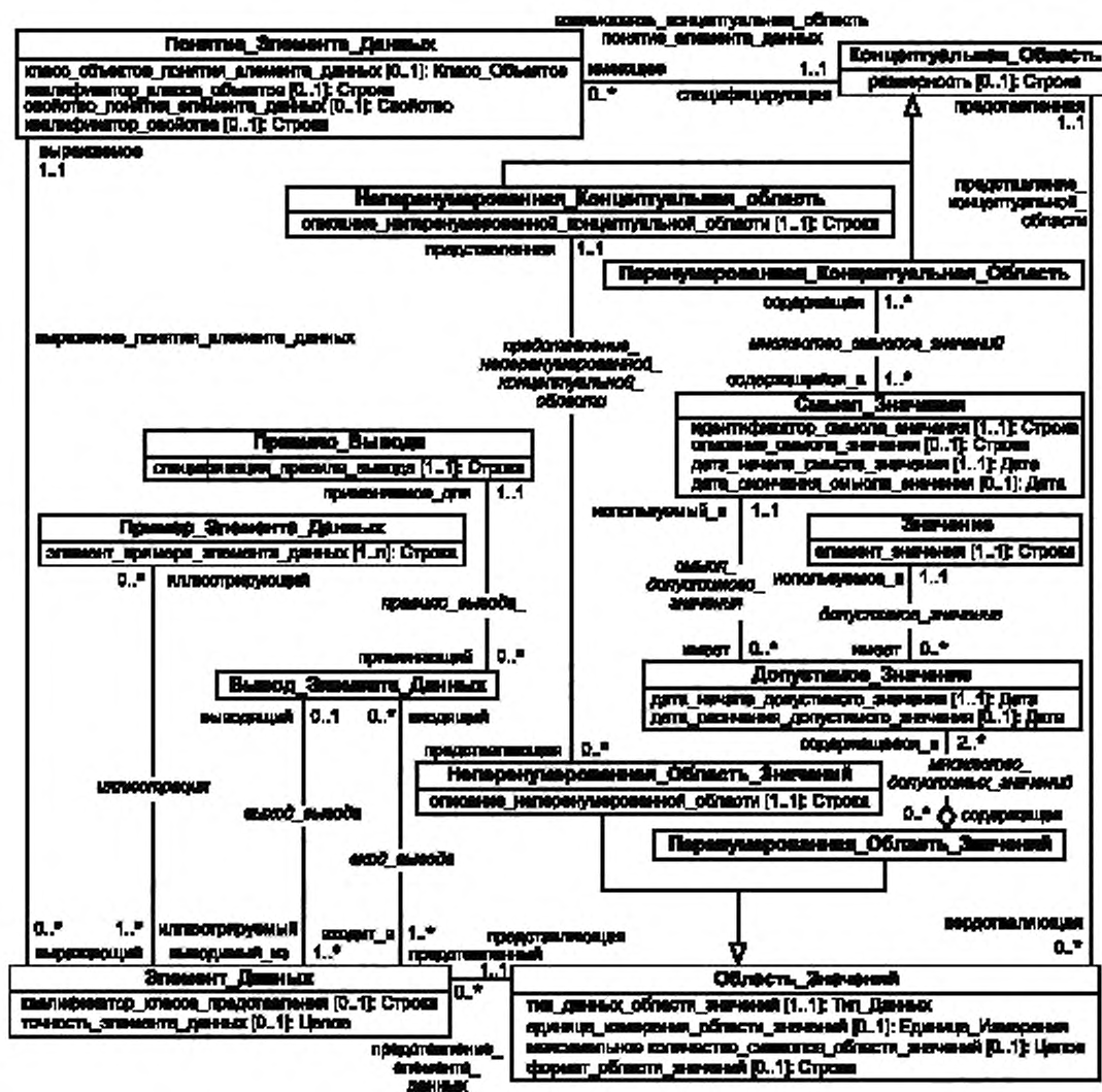
Рисунок 11 — Консолидированная метамодель
