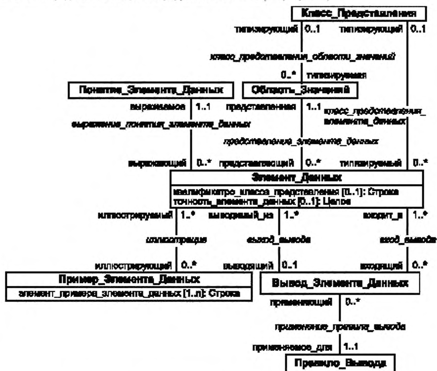
Рисунок 10 — Область метамодели, представляющая Элемент данных (Cor.1:2004)
