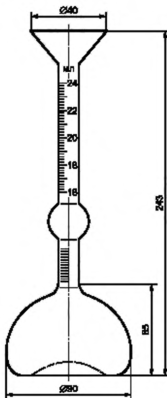
Рисунок 1 — Прибор Ле-Шателье
