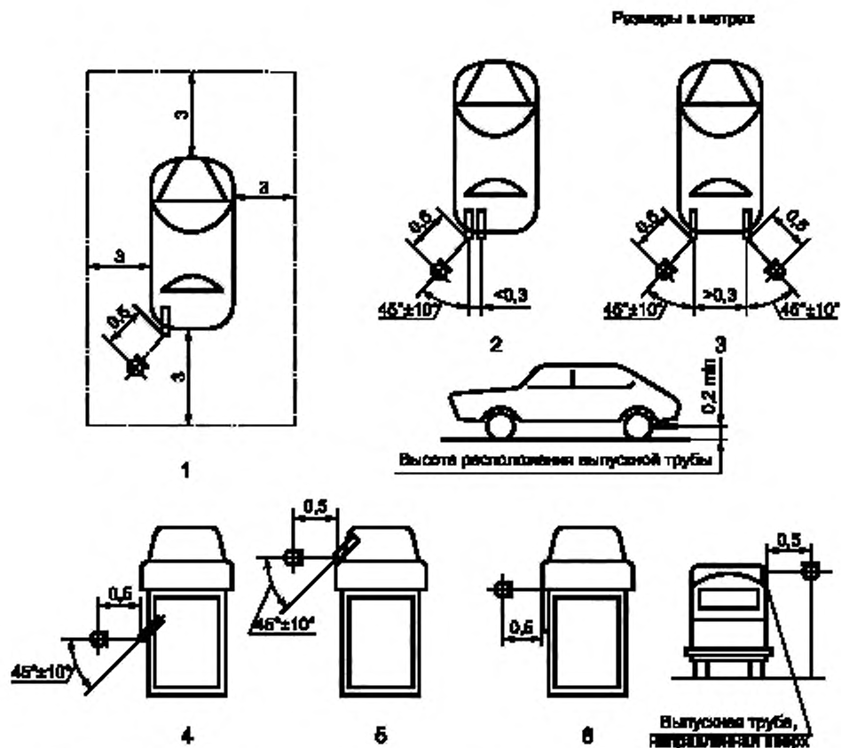
Рисунок Г.2 — Положения для измерений на автотранспортных средствах в неподвижном состоянии (примеры)
