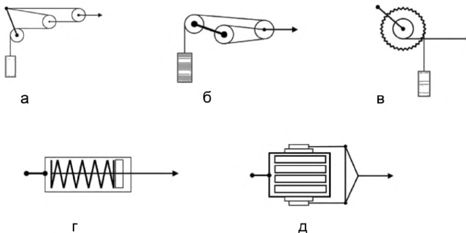
а — блочный; б — блочно-полиспастный; в — барабанный; г — пружинный с продольным расположением пружин; д — пружинный с поперечным расположением пружин
