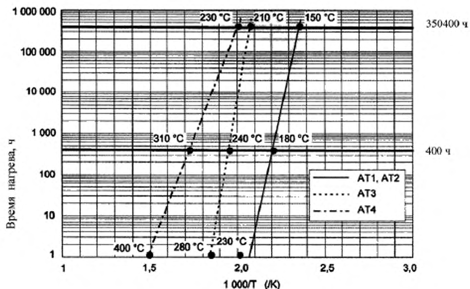
Рисунок А.1 — График Аррениуса (остаточное напряжение 90 %)
