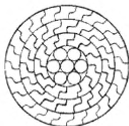
б) трехповивный провод, скрученный из профилированных проволок типа АхF/Sxy
