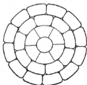
Рисунок 2 — Двухповивный провод, скрученный из профилированных проволок типа АхF/АуF
