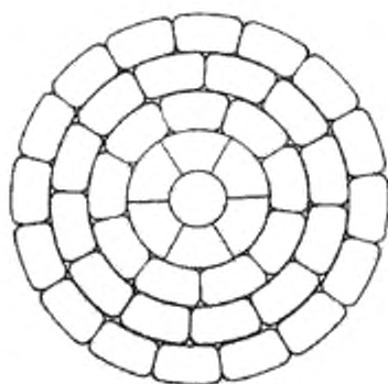
а) трехповивный провод, скрученный из профилированных проволок типа АхF/Sxy
