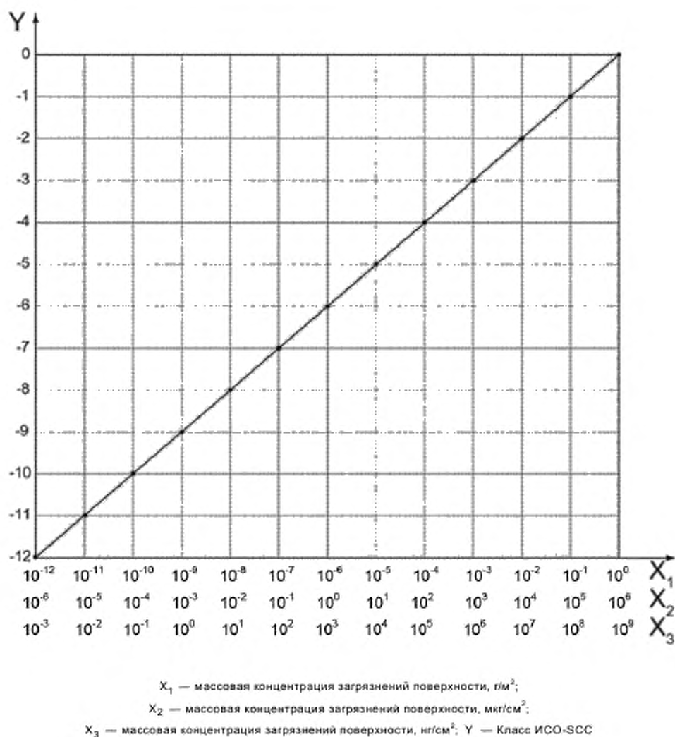
Рисунок 1 — Классы ИСО-SCC как функция концентрации загрязнений
