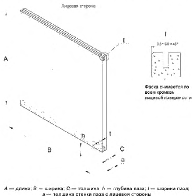
Рисунок 1 — Вид плиты под установку скрытым способом
