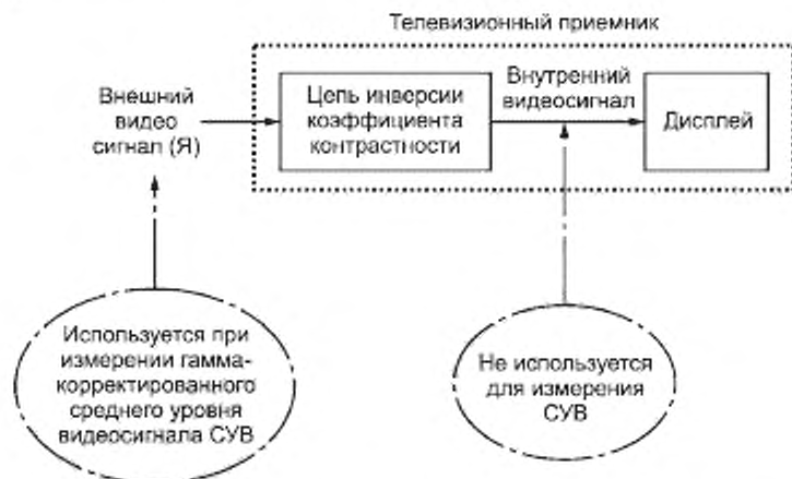
Рисунок 1 — Гамма-корректированный средний графический уровень
