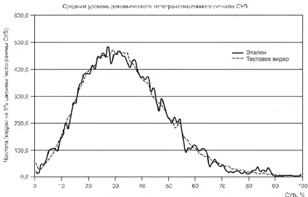
Рисунок С.1 — Средний уровень динамического теле трансляционного видеосигнала
