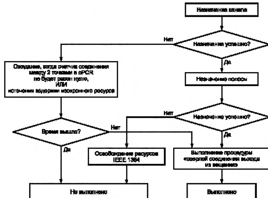
Рисунок 27 — Восстановление соединения выхода из вещания
