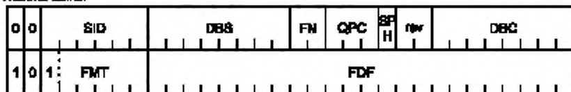
Рисунок 5 — Двухквადлетный CIP заголовок (form_0, form_1 = 0)
