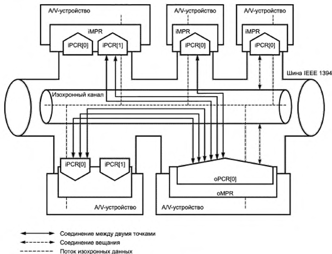
Рисунок 8 — Соединения
