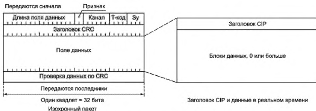
Рисунок 2 — Изохронный пакет
