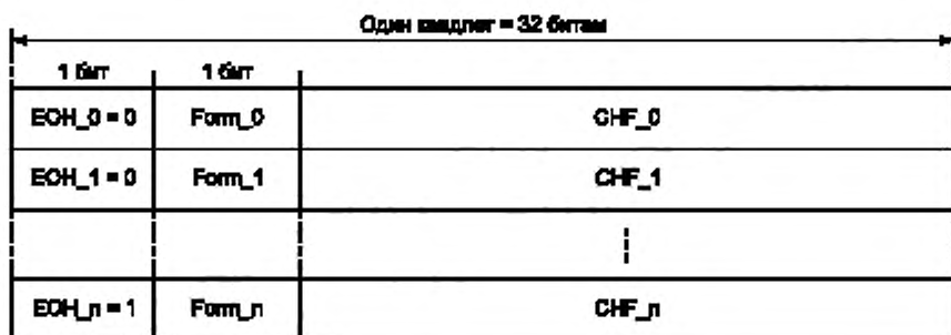
Рисунок 3 — Заголовок CIP
