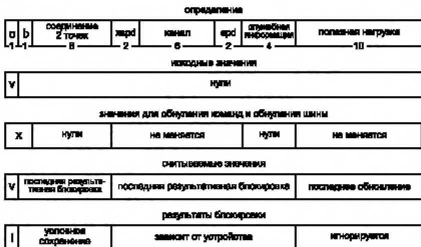
Рисунок 12 — Формат oPCR
