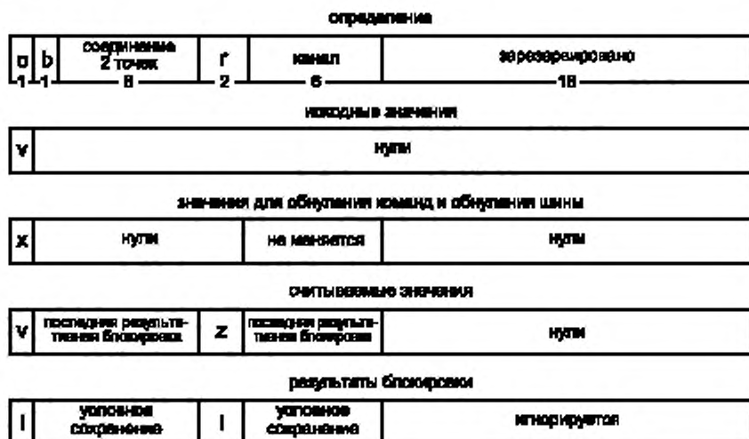
Рисунок 13 — Формат iPCR
