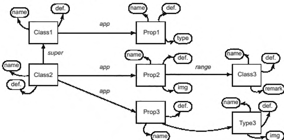
Рисунок E.5 — Результаты запрашивания объекта get_concept_model , пример 4
