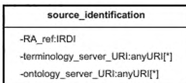
Рисунок 8 — Диаграмма класса UML для модели службы размещения
