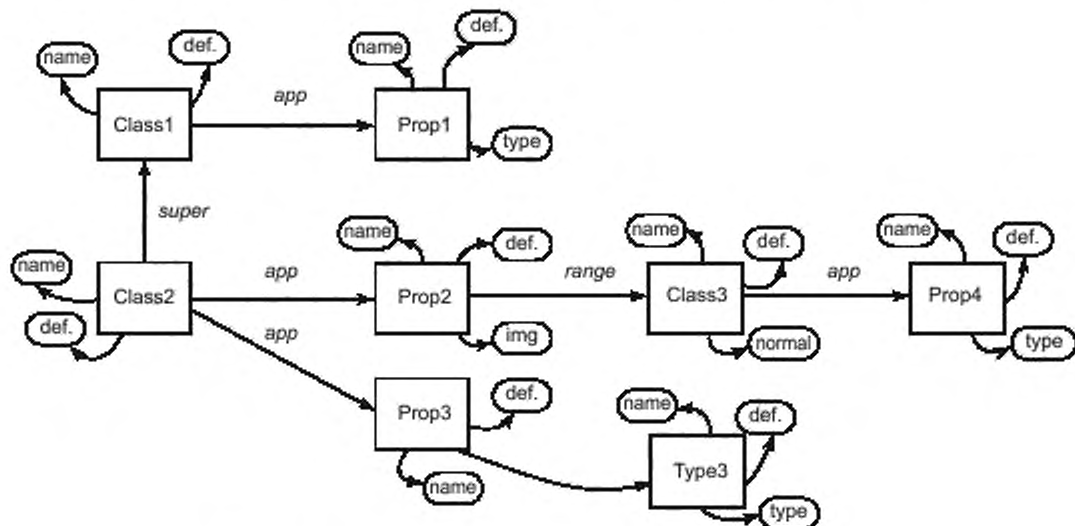
Рисунок E.1 — Определения и взаимоотношения онтологических концепций: экземпляр диаграммы
