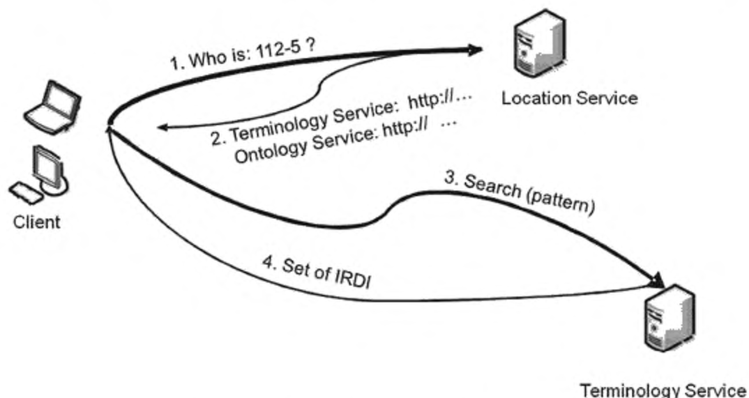
Рисунок 4 — Пример поиска концепций на Уровне 2
