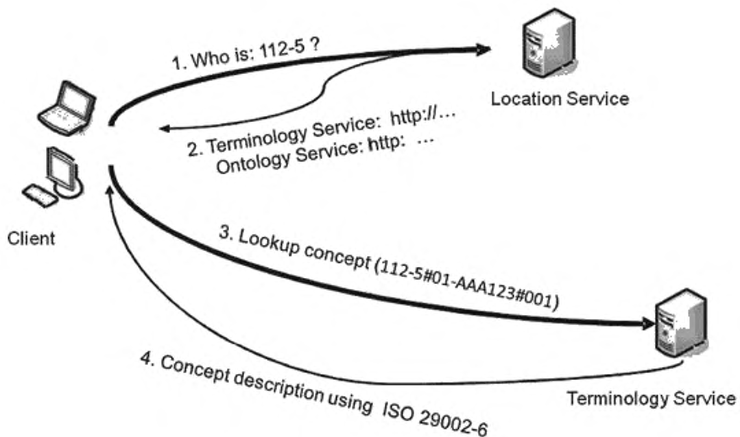
Рисунок 5 — Пример поиска концепций по идентификатору на Уровне 2
