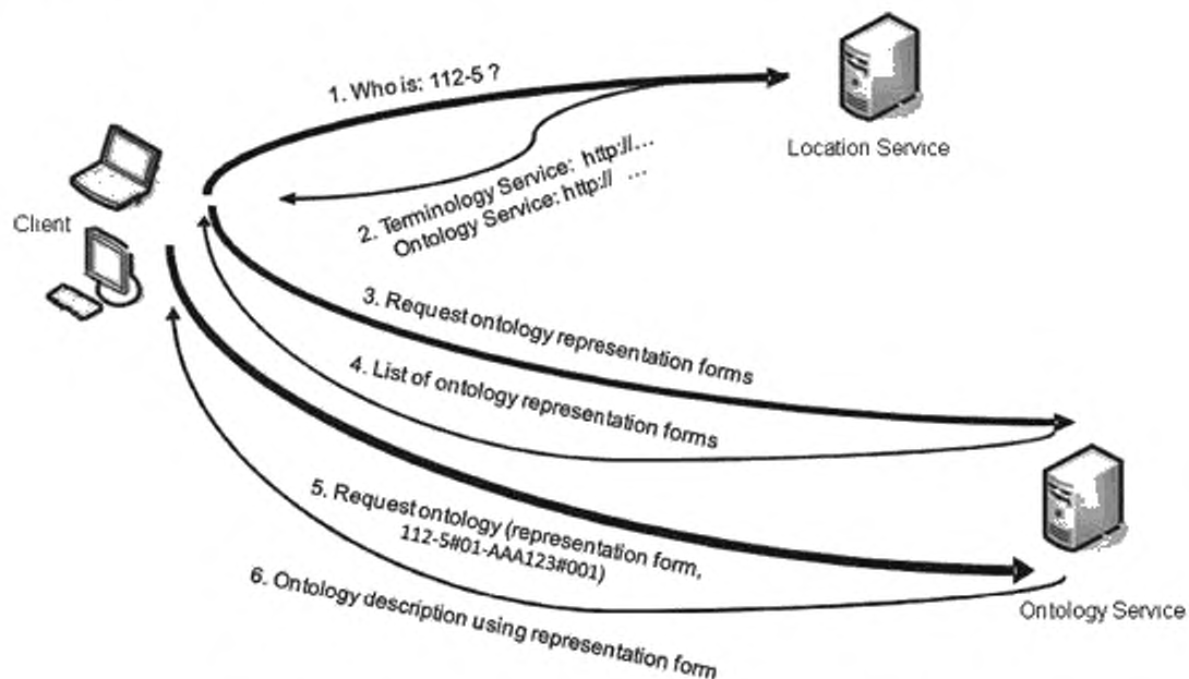
Рисунок 6 — Пример выборки онтологической информации на Уровне 3
