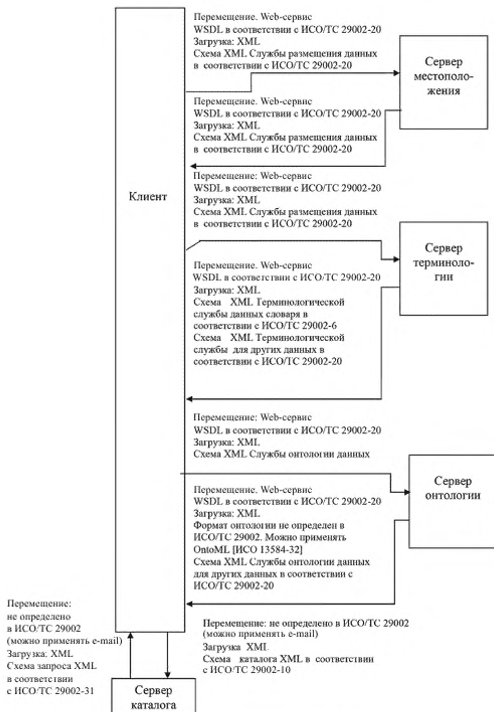
Рисунок 3 — Главные информационные потоки
