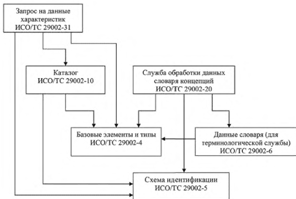
Рисунок 2 — Диаграмма зависимости частей и уровней
