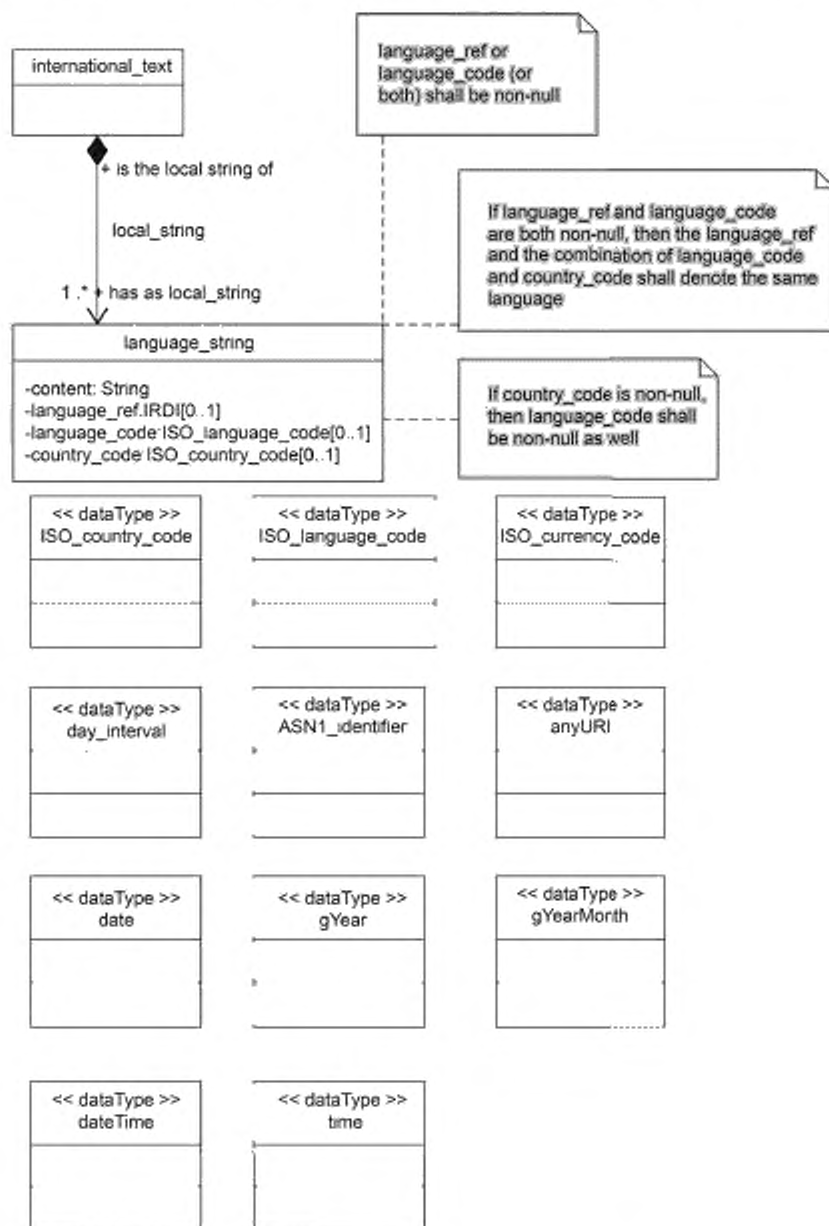
Рисунок 4 — Диаграмма класса UML для базовой модели данных
