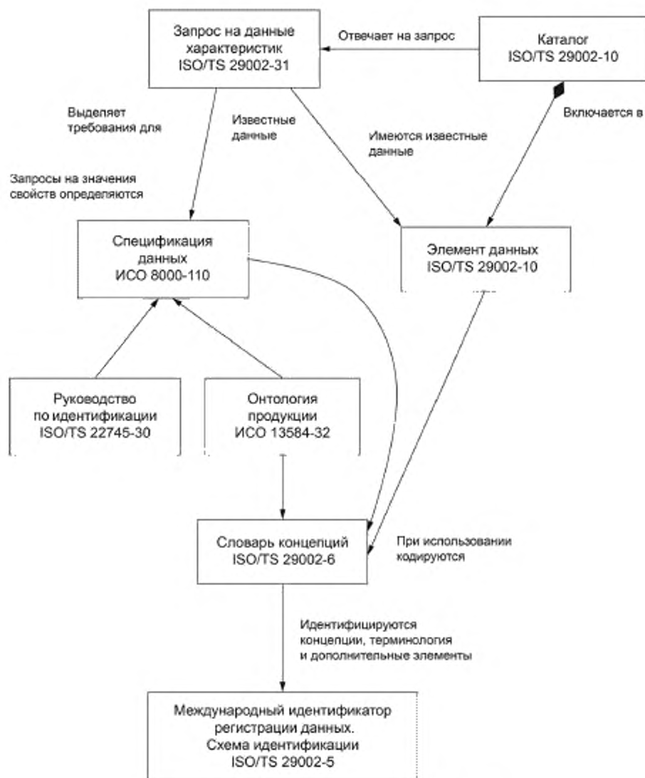
Рисунок 1 — Модель планирования высокого уровня
