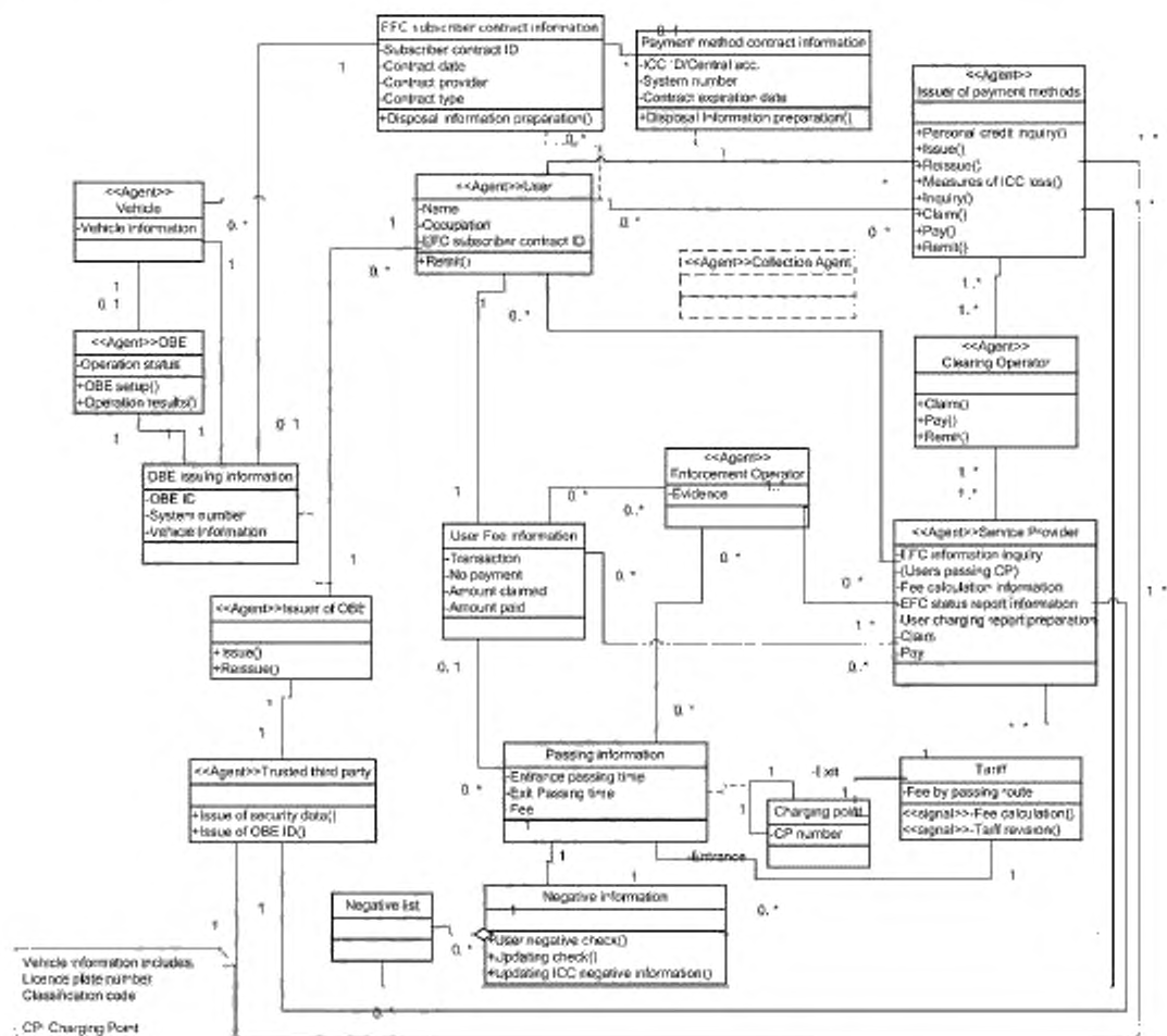
Рисунок E.1 — Пример диаграммы классов уведомления UML для сбора платежей
