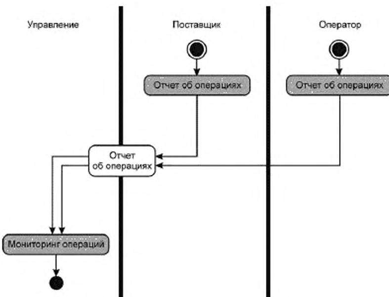
Рисунок 13 — Мониторинг операций
