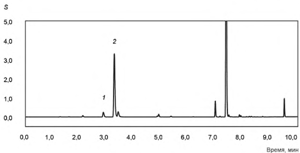
Рисунок В.3 — Хроматограмма концентрированного грейпфрутового сока, содержащего 48 \text{ млн}^{-1} метанола, с добавлением 0,01 % по массе внутреннего стандарта
