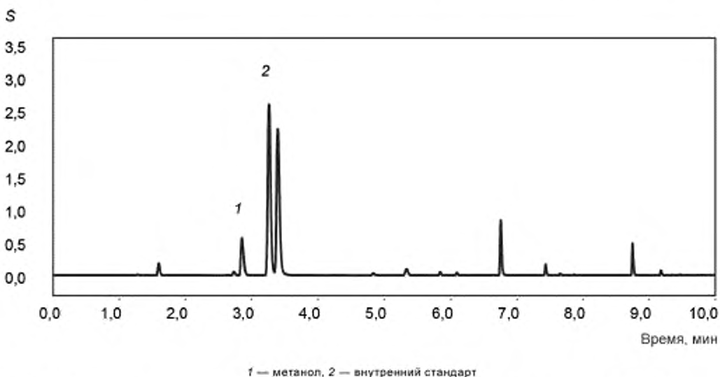
Рисунок В.2 — Хроматограмма осветленного яблочного сока прямого отжима, содержащего 160 \text{ млн}^{-1} метанола, с добавлением 0,01 % по массе внутреннего стандарта
