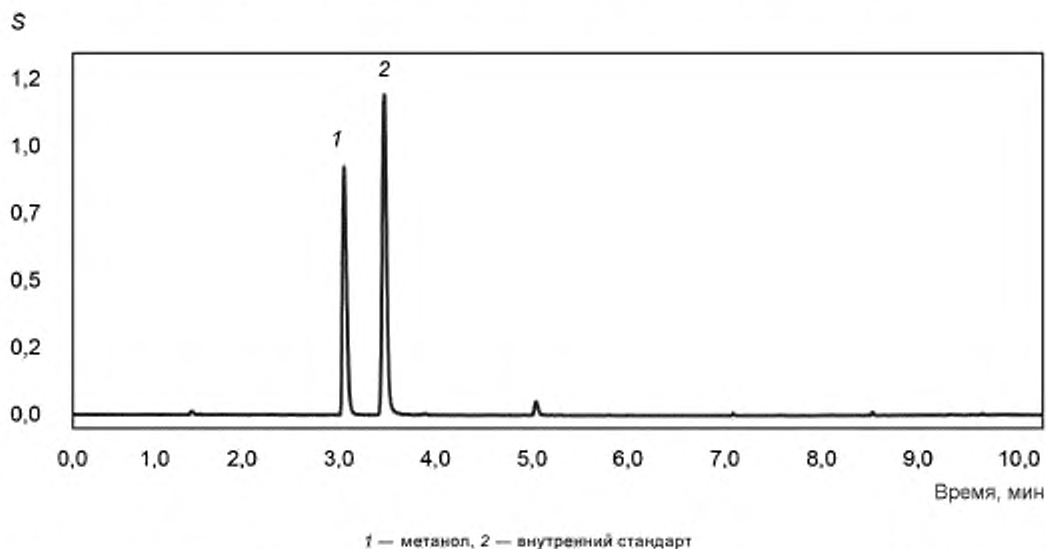
Рисунок В.1 — Хроматограмма градуировочного раствора, содержащего 250 \text{ млн}^{-1} метанола с добавлением 0,01 % по массе внутреннего стандарта
