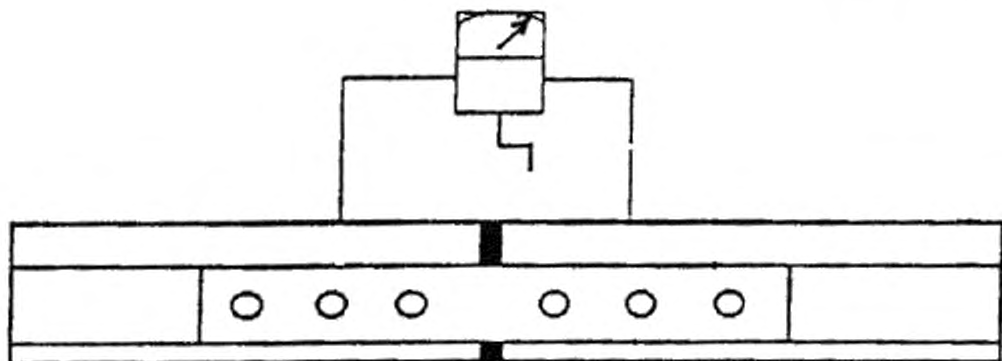
Рисунок 1 — Общая схема измерения электрического сопротивления изолирующего стыка
