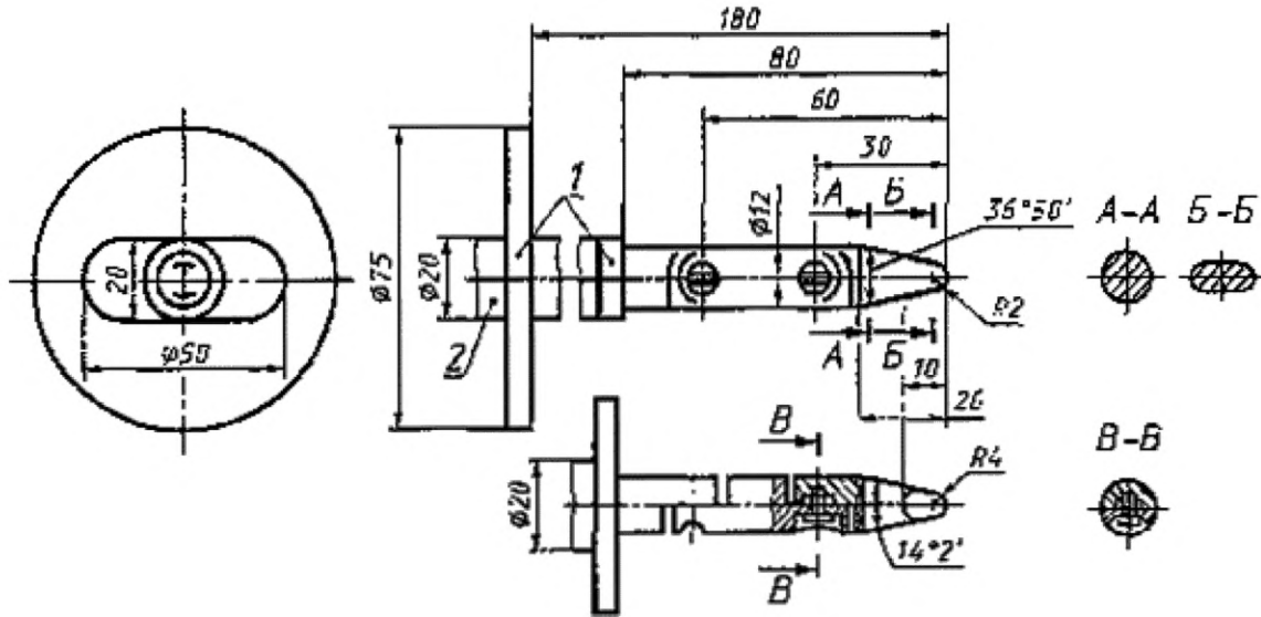
1 — ограничительные изоляционные бортики; 2 — ручка
