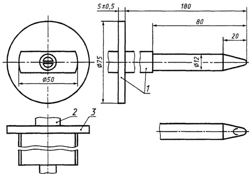
1 — изолирующий материал; 2 — рукоятка; 3 — ограничитель
