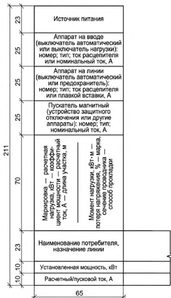
Ф о р м а 5 — Боковик принципиальной схемы магистрального и группового щитка освещения
