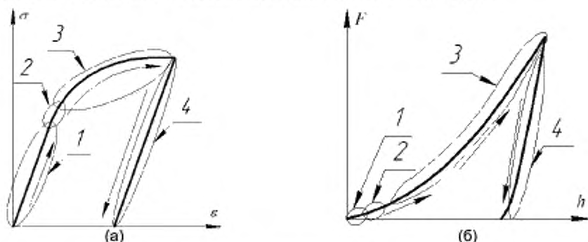
Рисунок Е.1 Схематичное изображение диаграмм: (а)растяжения, (б)вдавливании сферического индентора.
