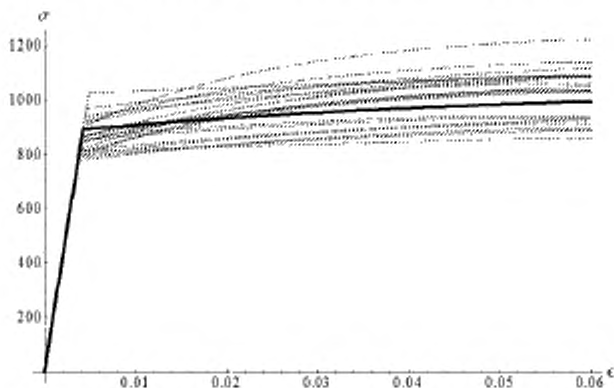
Рисунок Д.3 - Пример базы диаграмм растяжения со случайными отклонениями параметров для одного из состояний стали 15X2НМФА (сплошной линией обозначена аппроксимация экспериментально полученной диаграммы)
