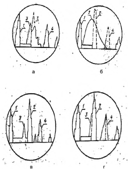
Рисунок В.1— Вид эхо-сигналов на экране дефектоскопа
