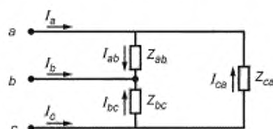
a, b, c — фазы основной вторичной обмотки ТН; I_a, I_b, I_c — фазные токи; I_{ab}, I_{bc}, I_{ca} — междофазные токи; Z_{ab}, Z_{bc}, Z_{ca} — междофазные нагрузки
