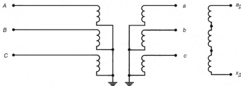
A, B, C — фазы первичной обмотки ТН; a, b, c — фазы основной вторичной обмотки ТН; xД — фазы дополнительной вторичной обмотки ТН
