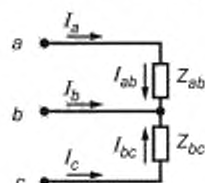
a, b, c — фазы основной вторичной обмотки ТН; I_a, I_b, I_c — фазные токи; I_{ab}, I_{bc} — междофазные токи; Z_{ab}, Z_{bc} — междофазные нагрузки
