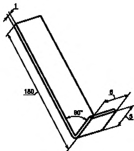
Рисунок PS-D.4 — Испытательный крюк
