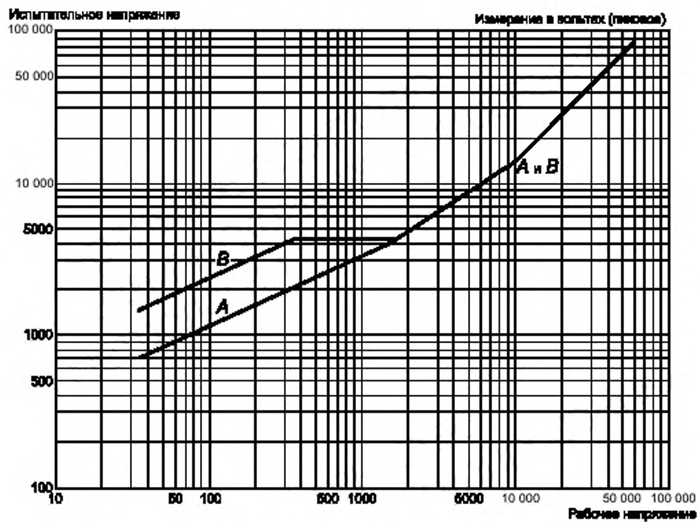
Рисунок PS-D.7 — Испытательные напряжения
