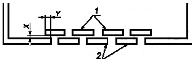
Y — 2 X, но не менее 25 мм; 1 — пластины отражателя (могут быть расположены под дном оболочки); 2 — дно оболочки
