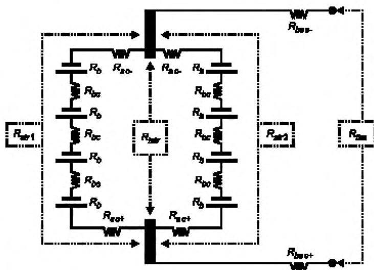
Рисунок PS-E.1.100.A — Расчеты сопротивления и короткого замыкания
