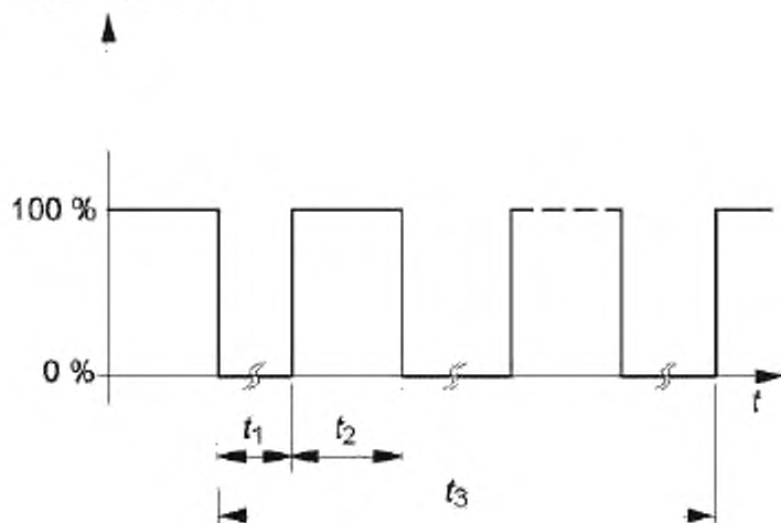
Рисунок L.2 – Питающее напряжение для функциональных испытаний
