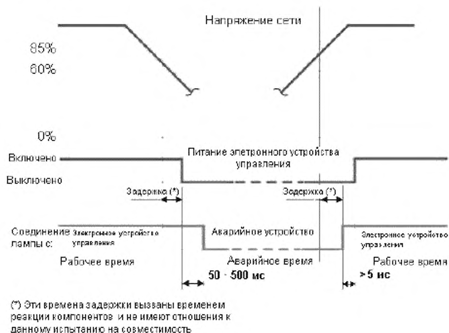
Рисунок L.1 – Временная диаграмма операции переключения
