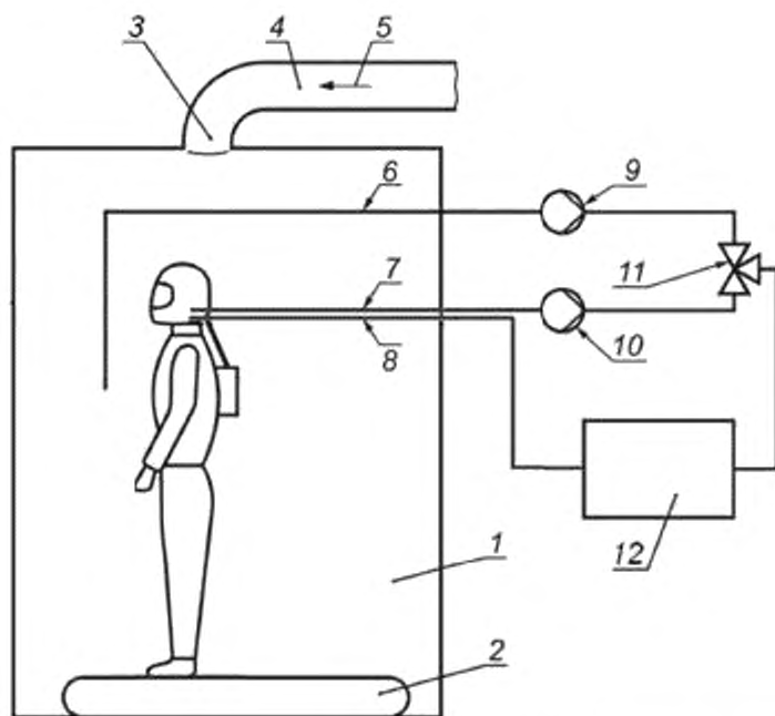
1 — камера; 2 — беговая дорожка; 3 — заслонка; 4 — труба; 5 — воздух + SF_6 ; 6 — линия пробоотбора в камере; 7 — линия пробоотбора в дыхательной зоне; 8 — линия возврата пробы в дыхательную зону; 9, 10 — насосы для отбора проб; 11 — переключающий клапан; 12 — анализатор
