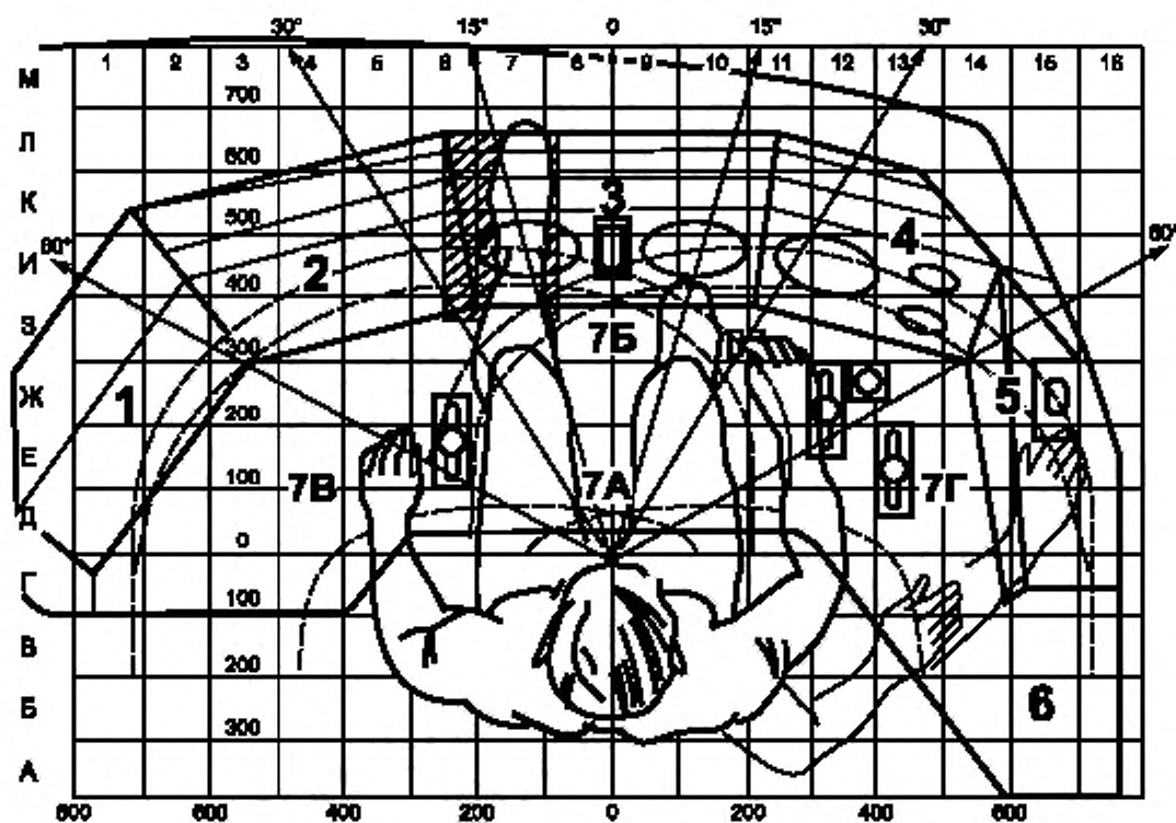
Рисунок А.1 — Компонка СОИ и ОУ
