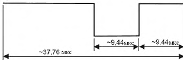
Рисунок 9 – Конец кадра при любом способе кодирования
