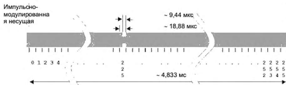
Рисунок 3 – Способ кодирования «1 из 256»
