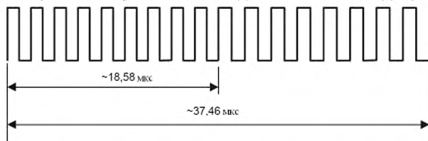
Рисунок 13 – Логическая единица при использовании двух поднесущих
