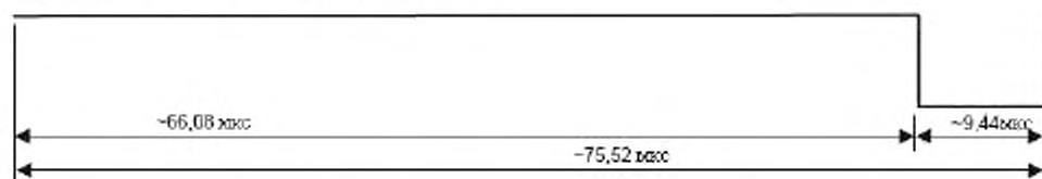
Рисунок 5 – Способ кодирования «1 из 4»
