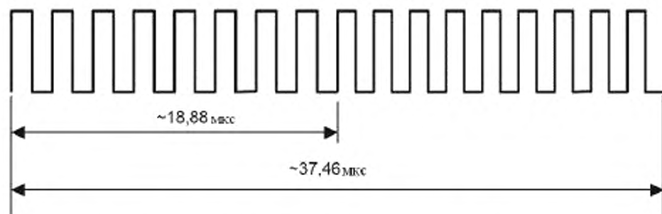
Рисунок 12 – Логический ноль при использовании двух поднесущих
