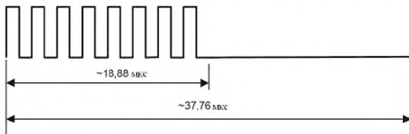
Рисунок 10 – Логический ноль
