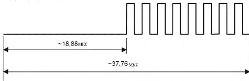
Рисунок 11 – Логическая единица
