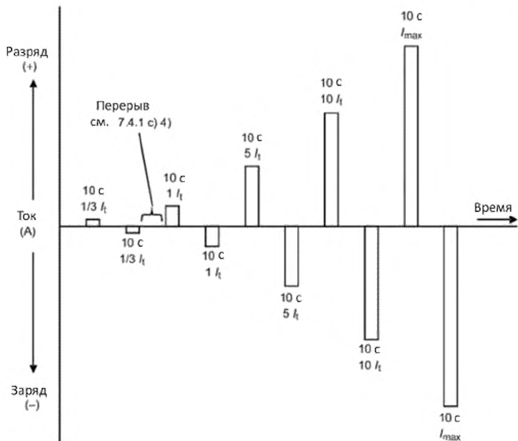
Рисунок 3, лист 1 — Порядок испытаний по определению вольт-амперных характеристик
