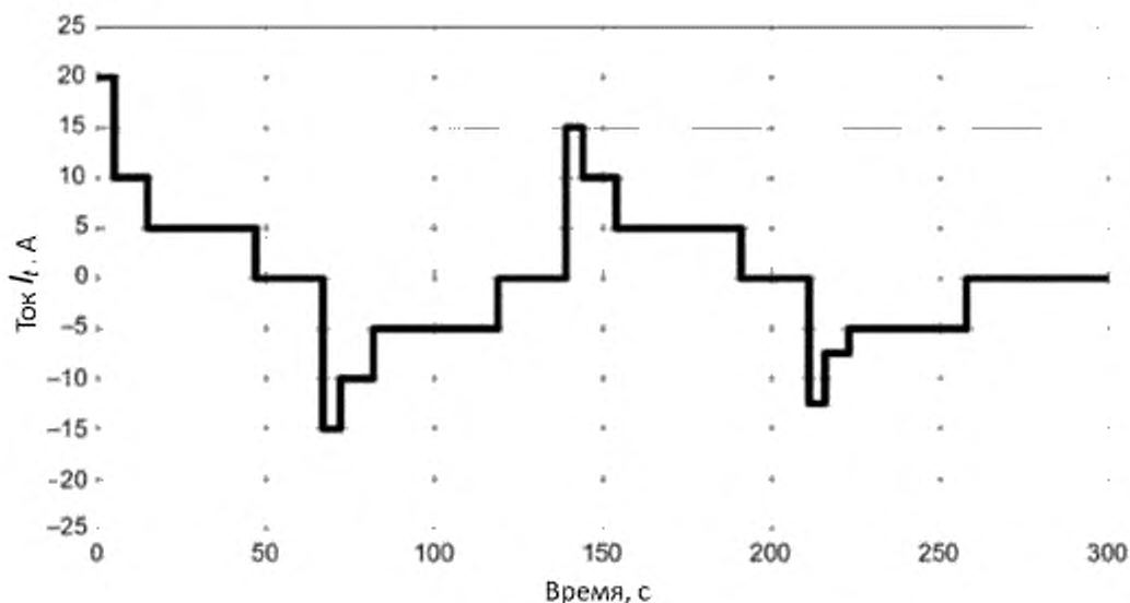
Рисунок 6 — ППЗ при циклировании аккумуляторов для ЭМГ
