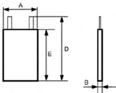
e – плоский аккумулятор (1)
