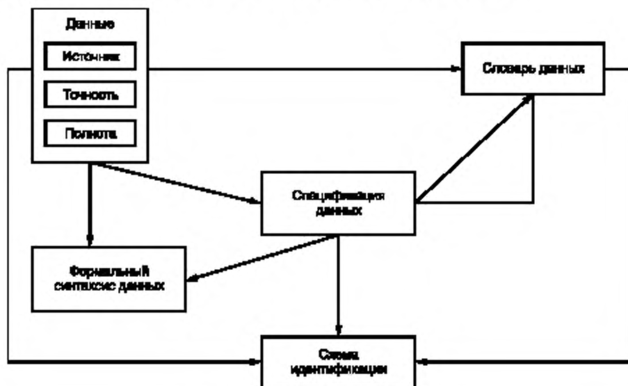
Рисунок 1 — Структура данных
